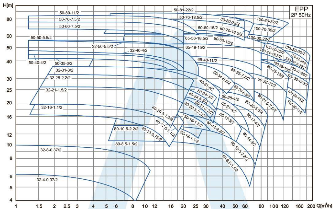
КРИВЫЕ ПРОИЗВОДИТЕЛЬНОСТИ
