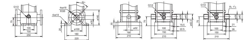
DIN фланец (EVR) Хомутное соединение (EVS) Резьбовое соединение (EVS)
