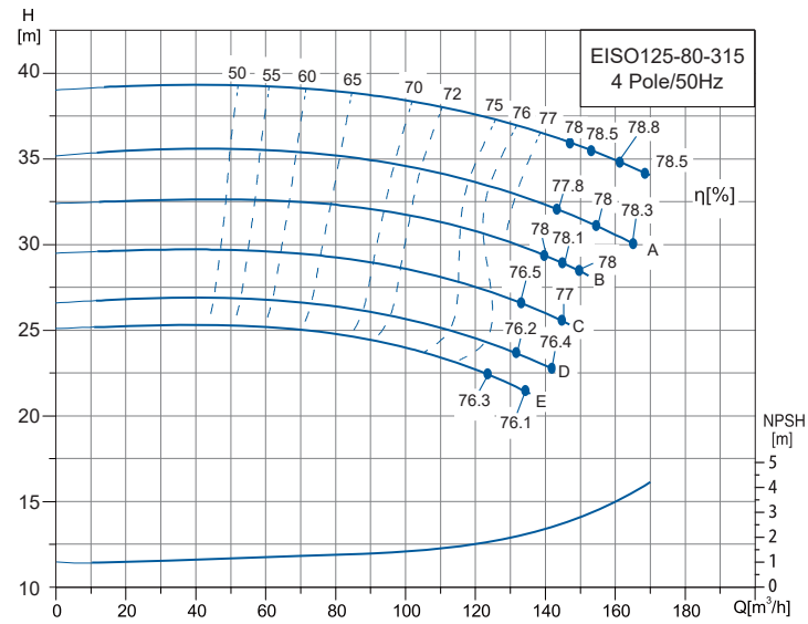
EISO125-80-315 1450 r/min
