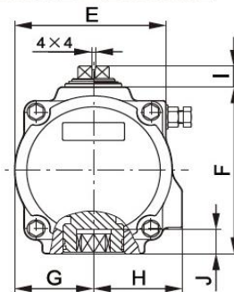
ISO5211 / VDI/VDE3845
