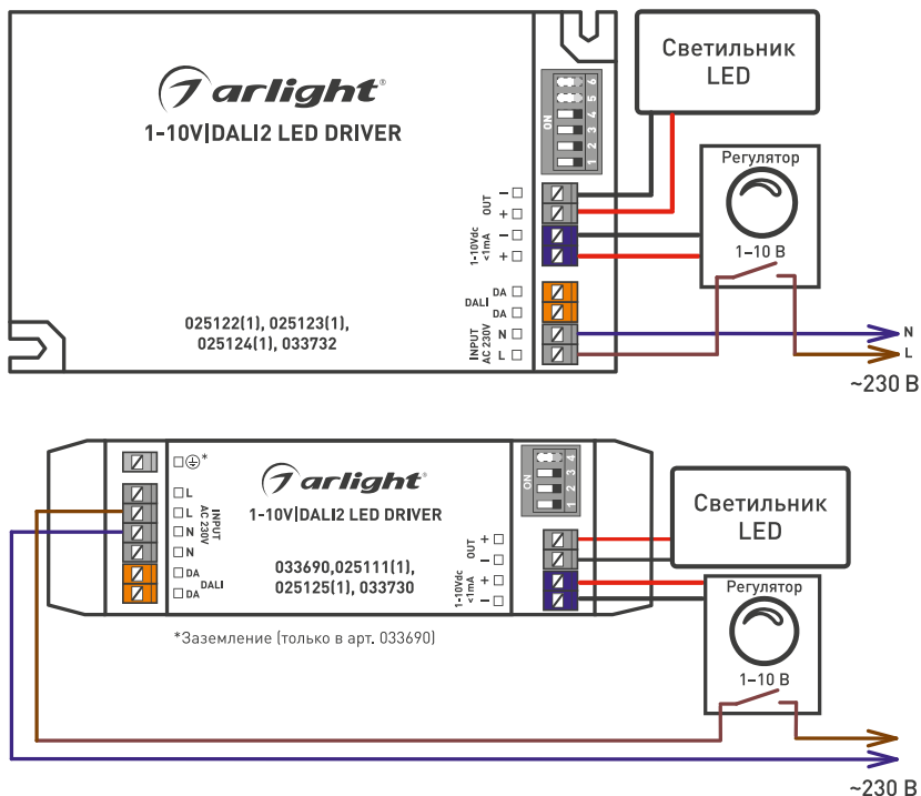
Рис. 3. Подключение источника тока при управлении регулятором 1-10 В
