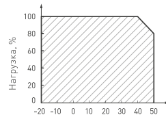
Температура окружающей среды (ta), °C Рис. 3. Максимальная допустимая нагрузка, % от мощности источника
