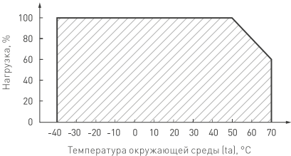
Рис. 2. Максимальная допустимая нагрузка, % от мощности источника
