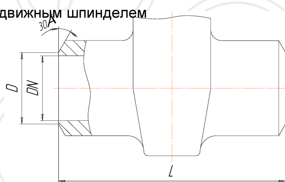
Рисунок 3. Исполнение под приварку
