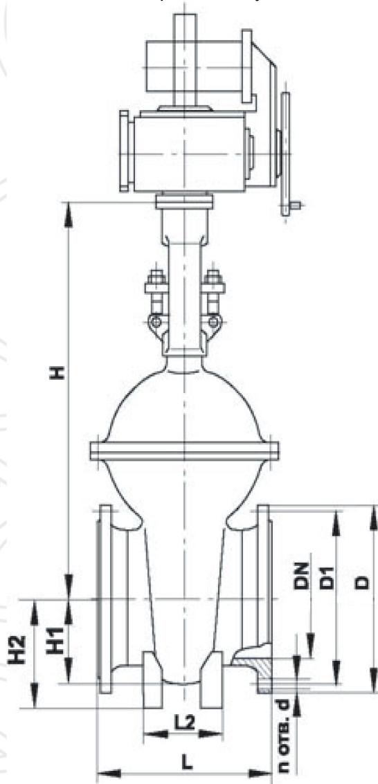
Рисунок 4. Задвижка с невымываемым шпинделем
