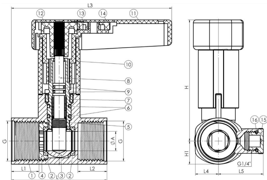
Рис.1 Клапан балансировочный ручной латунный без измерительных ниппелей.
