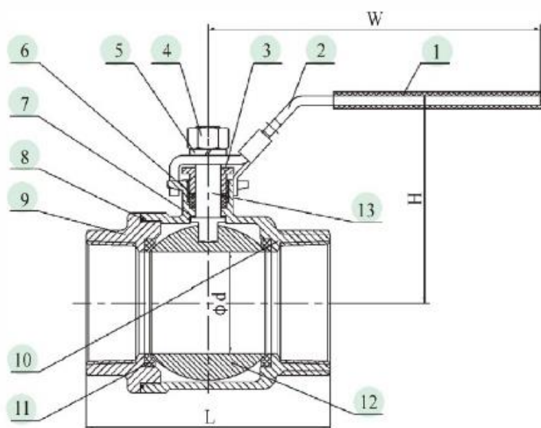
Рис. 1. Кран шаровой муфтовый.
