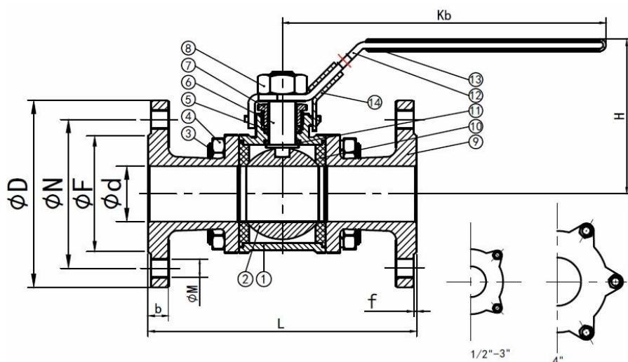
Рис.1 Кран трехсоставной шаровой фланцевый.
