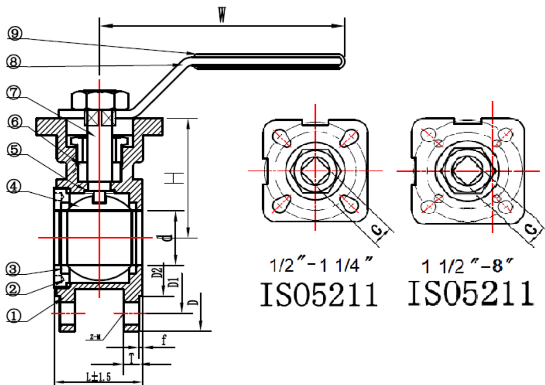
Рис.1 Кран шаровой межфланцевый.
