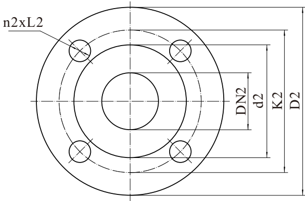
Патрубок нагнетания
