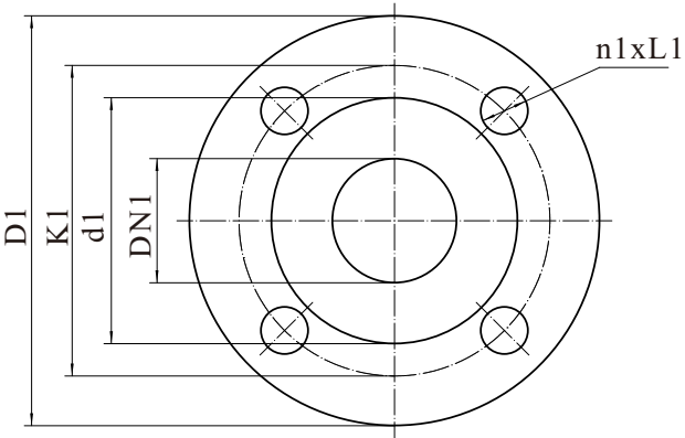
Патрубок всасывания
