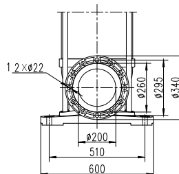
*Фланец PN16/DN200
