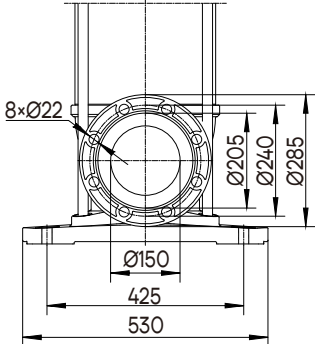
*Фланец PN16/DN150
