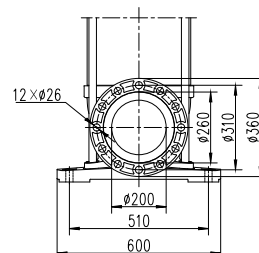
*Фланец PN25/DN200
