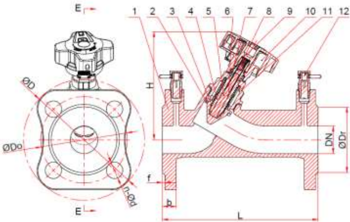
Габаритный чертеж клапана балансировочного Ду50-65
