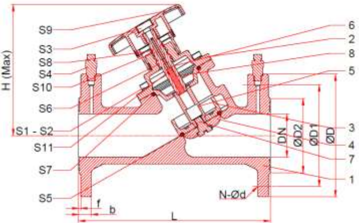
Габаритный чертеж клапана балансировочного Ду50-65
