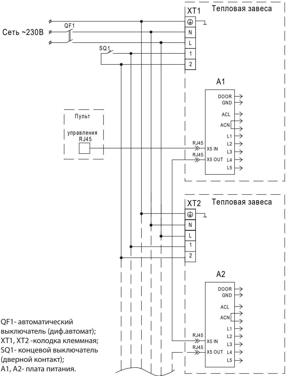
Рисунок 18. Принципиальная схема группового подключения завес к одному пульту управления KRC-14.
