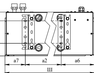
РАЗМЕРЫ КРОНШТЕЙНА
