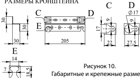
РАЗМЕРЫ КРОНШТЕЙНА
