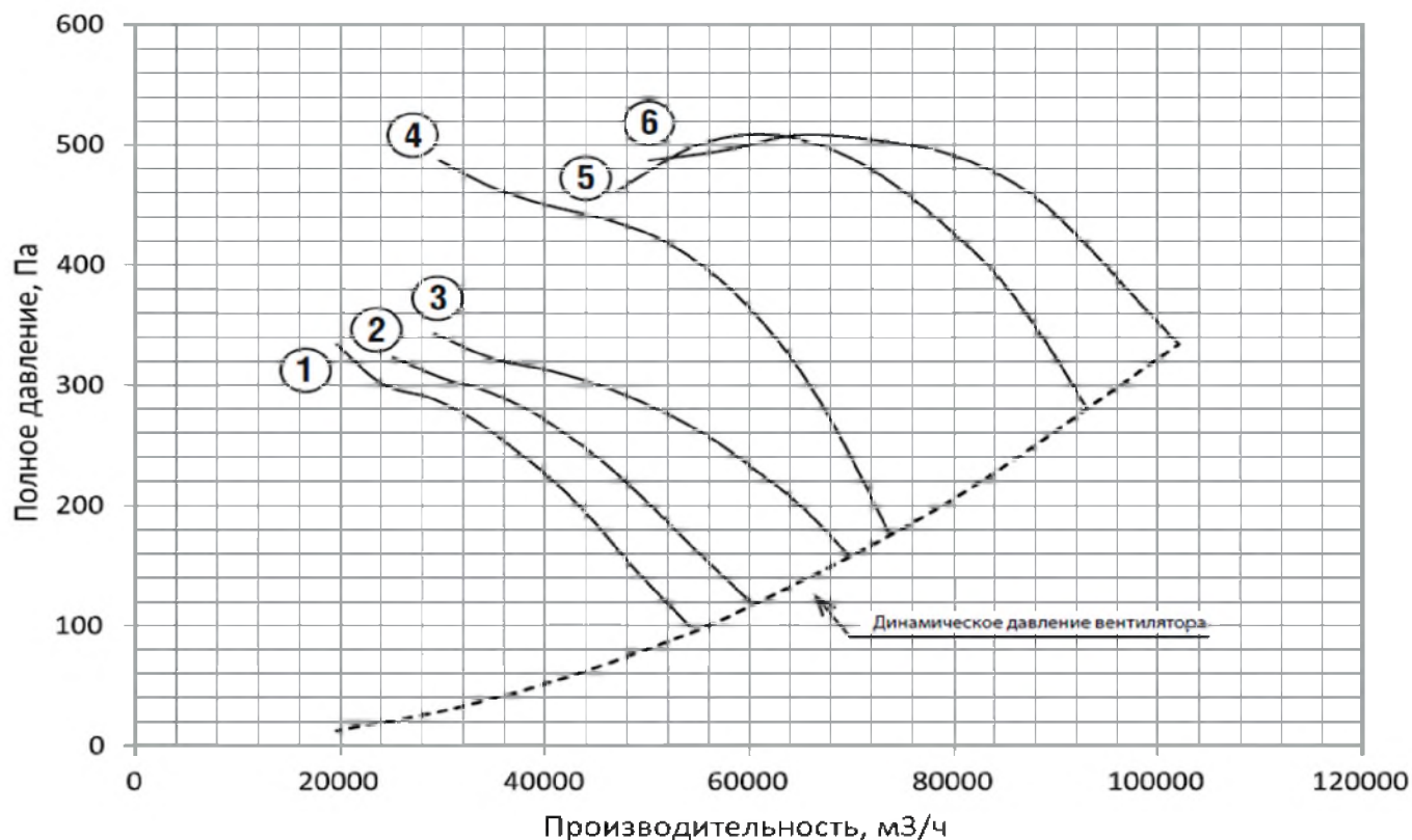
Рис. 13 Аэродинамическая характеристика AXIS TOP №12,5 1000 об/мин
