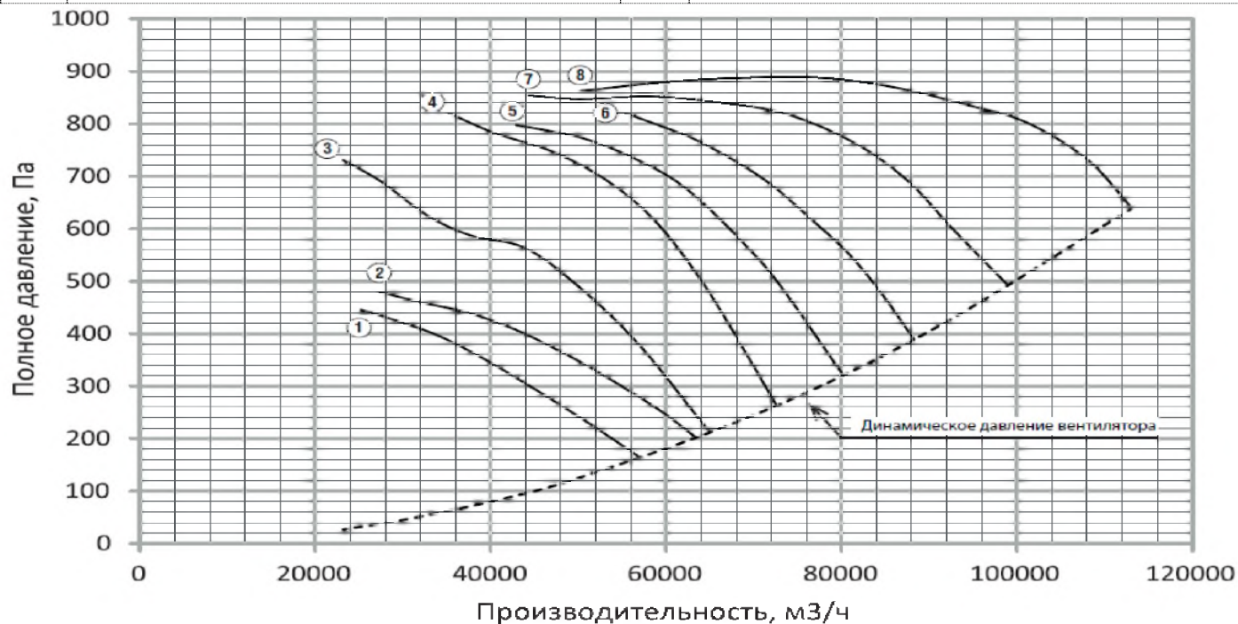
Рис 12. Аэродинамическая характеристика вентилятора AXIS TOP №11,2 1500 об/мин.
