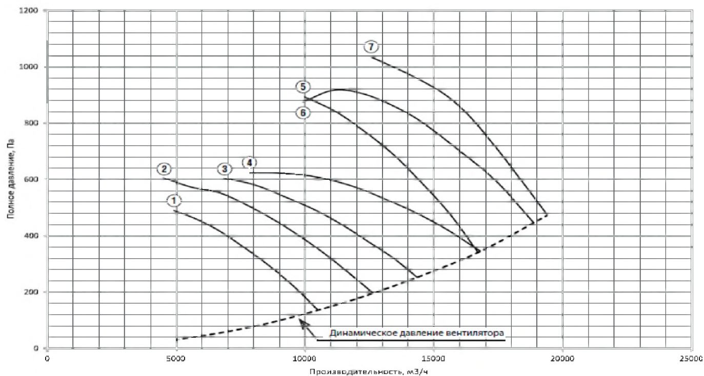
Рисунок 4. Аэродинамическая характеристика вентилятора AXIS TOP №5
