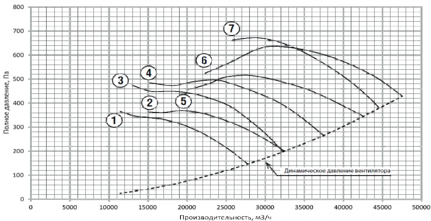
Рисунок 8. Аэродинамическая характеристика вентилятора AXIS TOP №8 1500 об/мин
