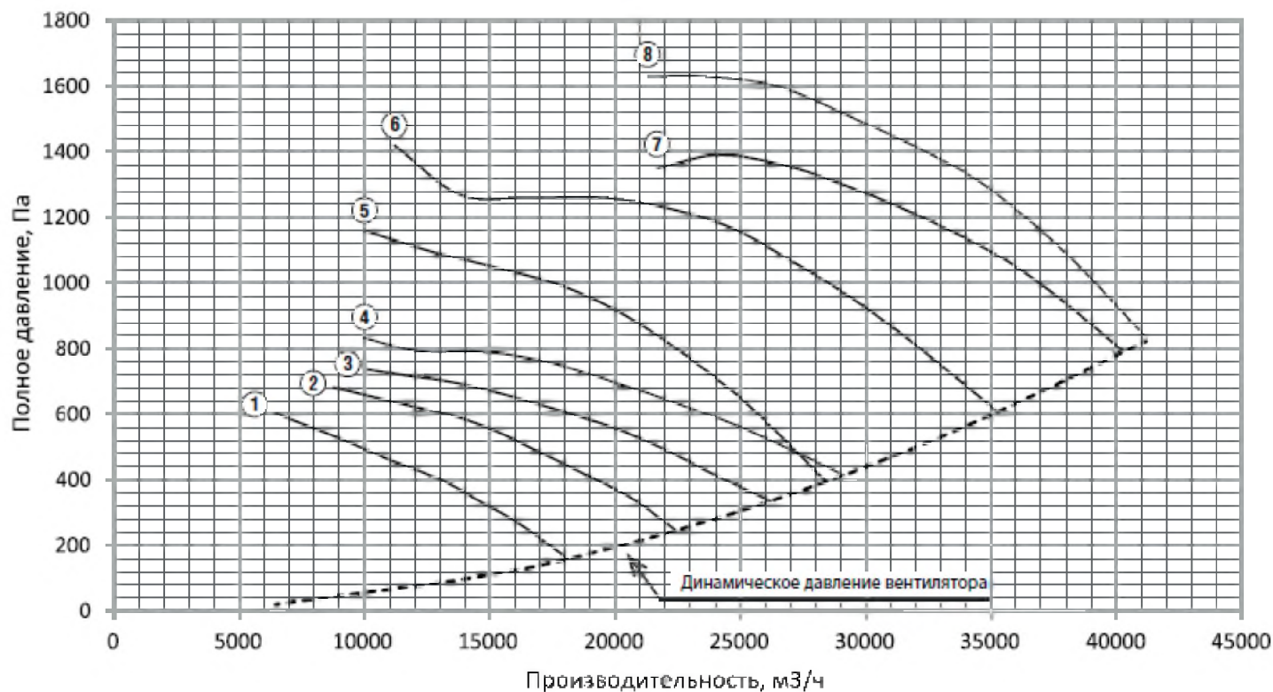
Рисунок 6. Аэродинамическая характеристика вентилятора AXIS TOP №6,3
