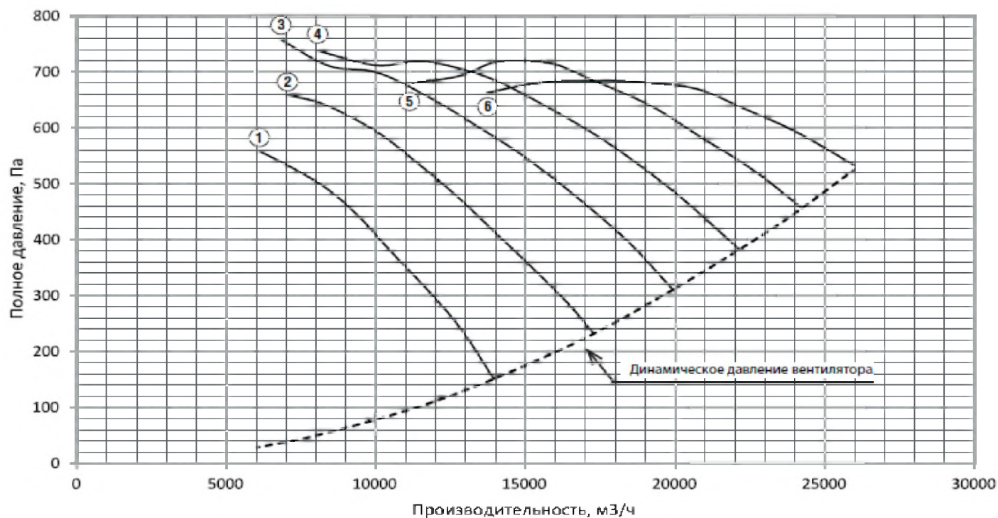
Рисунок 5. Аэродинамическая характеристика вентилятора AXIS TOP №5,6
