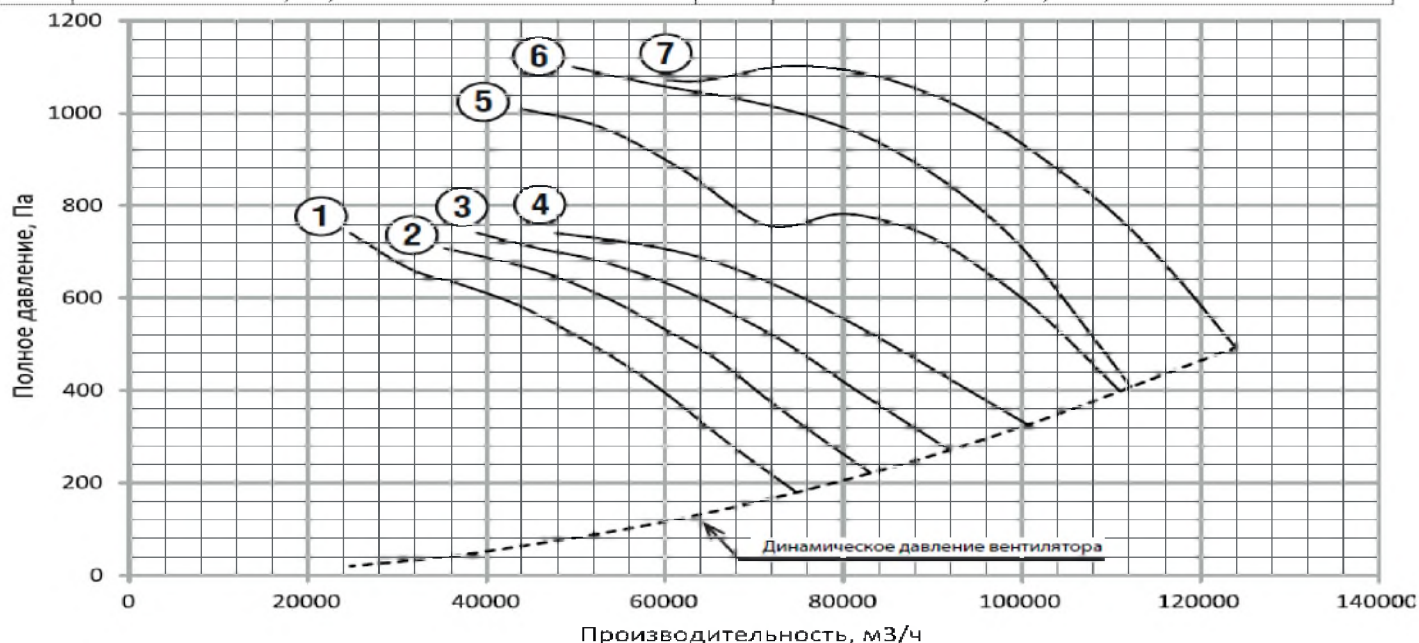
Рис. 14 Аэродинамическая характеристика AXIS TOP №12,5 1500 об/мин
