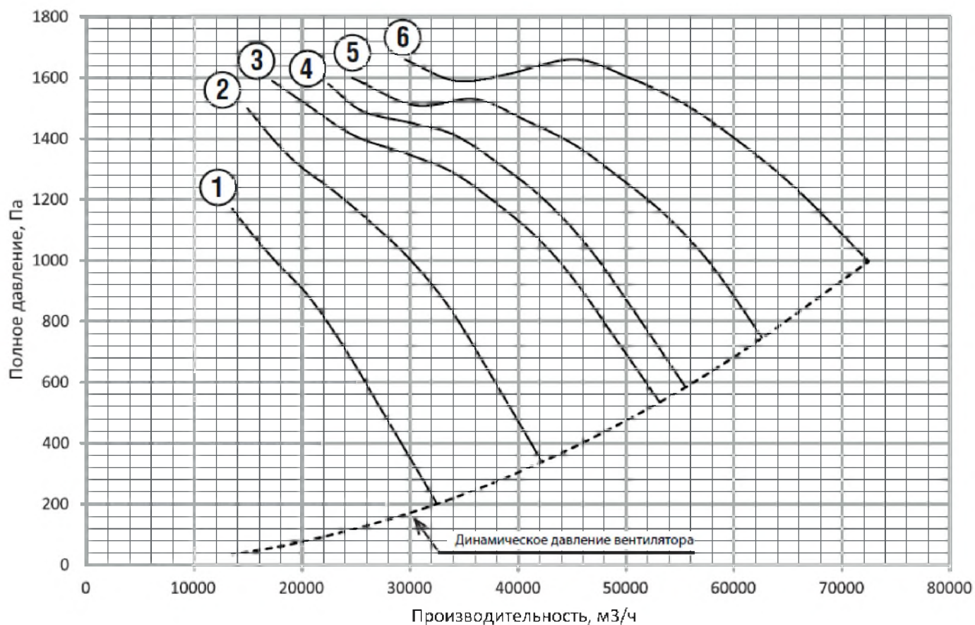
Рисунок 9. Аэродинамическая характеристика вентилятора AXIS TOP №8 3000 об/мин
