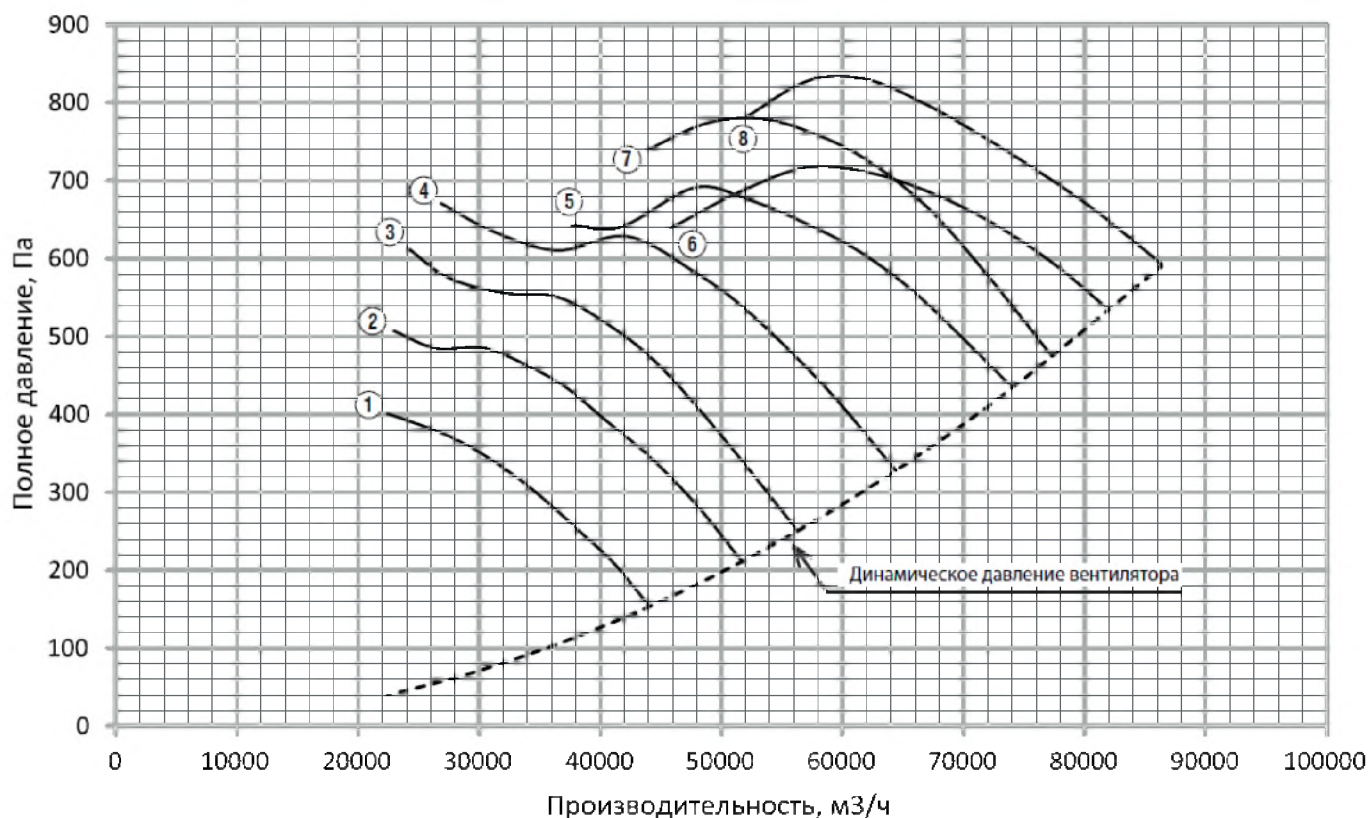
Рисунок 11. Аэродинамическая характеристика вентилятора AXIS TOP №10 1500 об/мин
