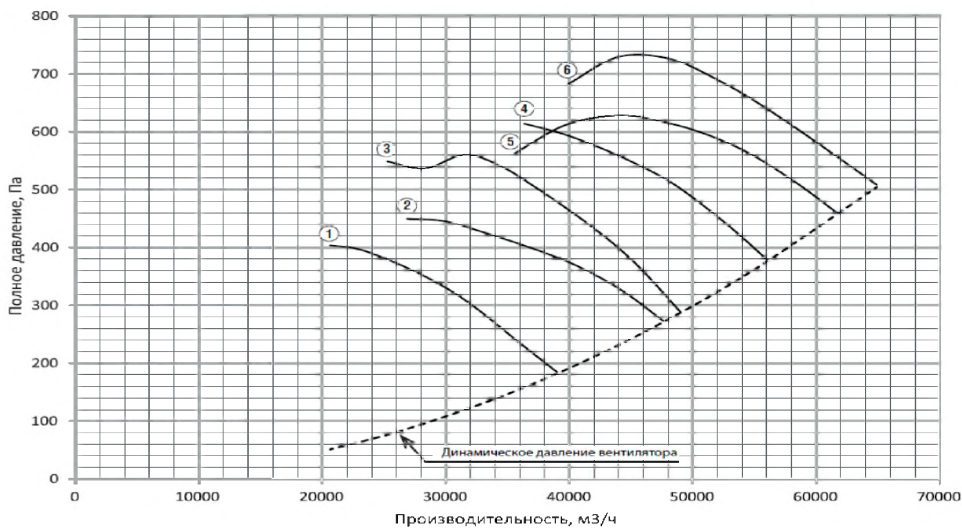
Рисунок 10. Аэродинамическая характеристика вентилятора AXIS TOP №9 1500 об/мин
