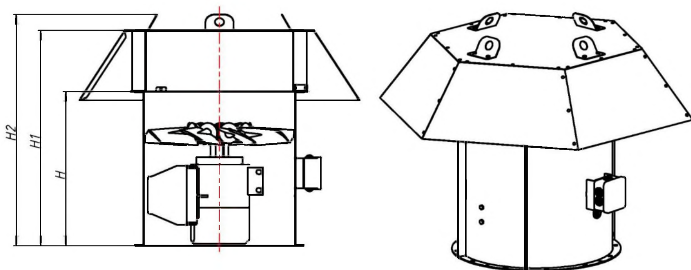
Рисунок 1. Габаритные и присоединительные размеры вентилятора
