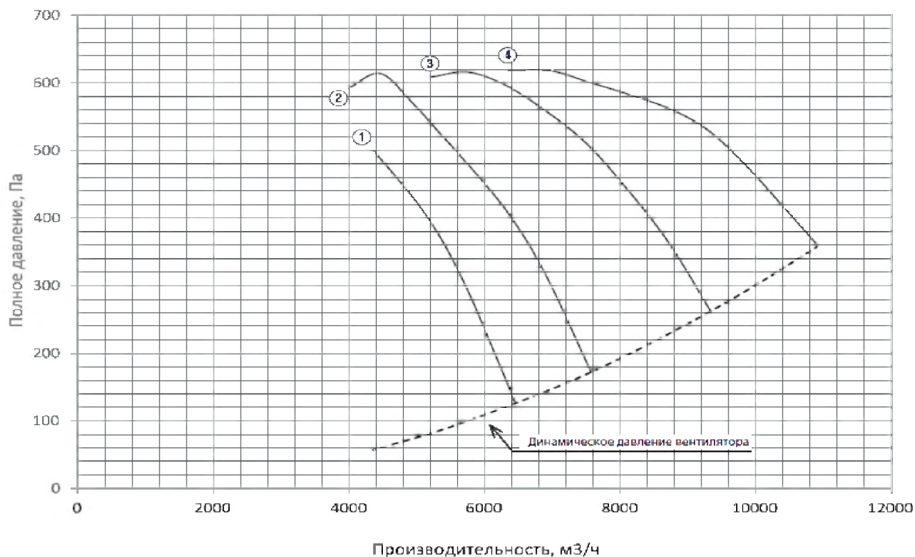
Рисунок 2. Аэродинамическая характеристика вентилятора AXIS TOP №4
