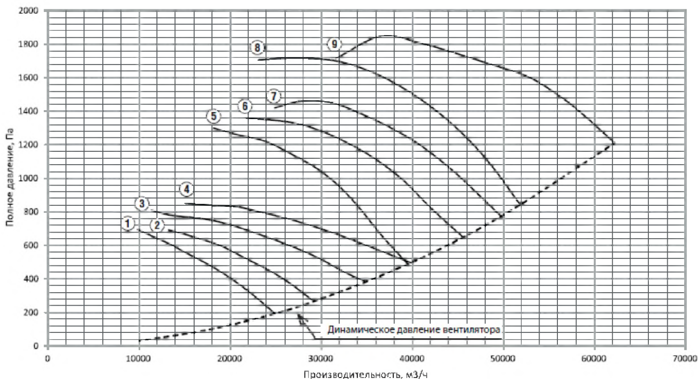
Рисунок 7. Аэродинамическая характеристика вентилятора AXIS TOP №7,1
