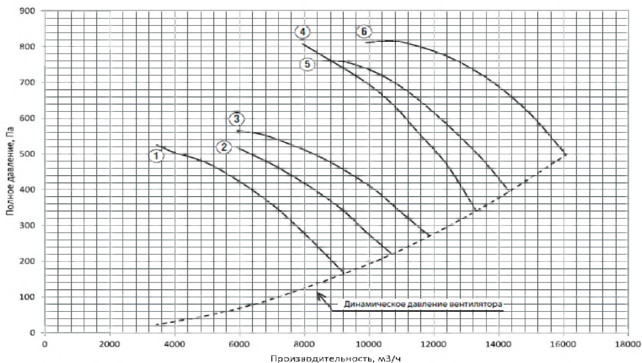
Рисунок 3. Аэродинамическая характеристика вентилятора AXIS TOP №4,5
