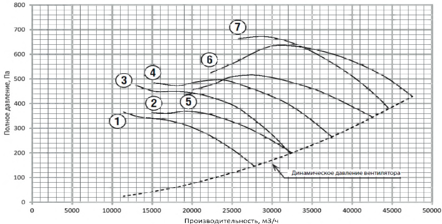
Рисунок 8. Аэродинамическая характеристика вентилятора AXIS №8 1500 об/мин
