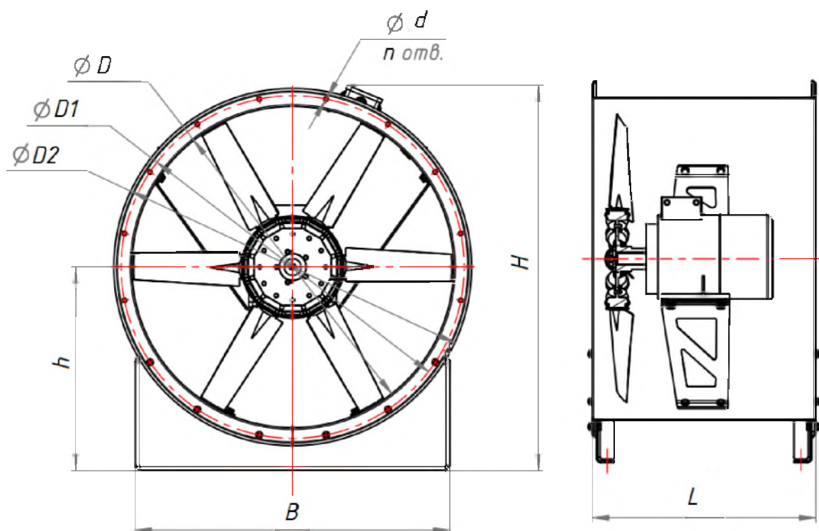
Рисунок 1. Габаритные и присоединительные размеры вентилятора
