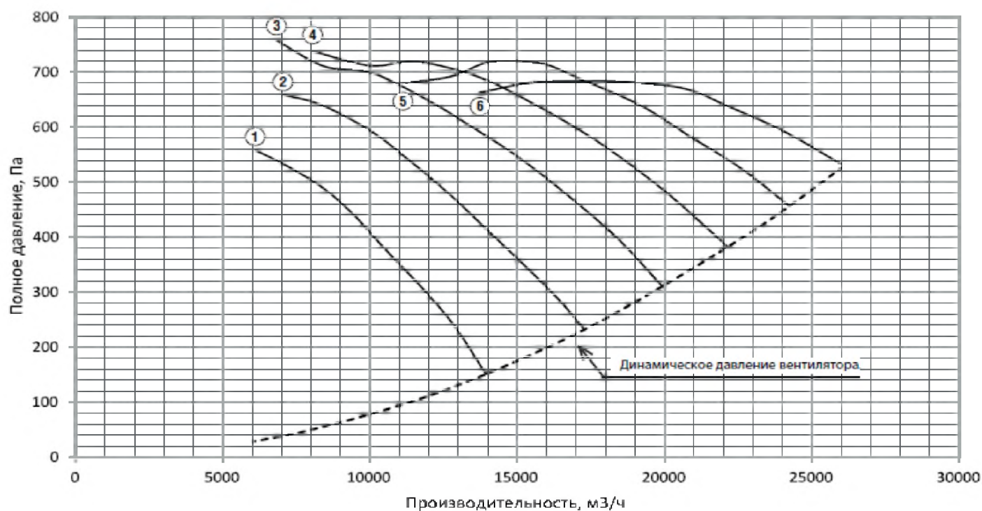
Рисунок 5. Аэродинамическая характеристика вентилятора AXIS №5,6
