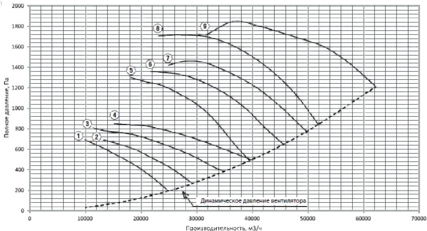
Рисунок 7. Аэродинамическая характеристика вентилятора AXIS №7,1
