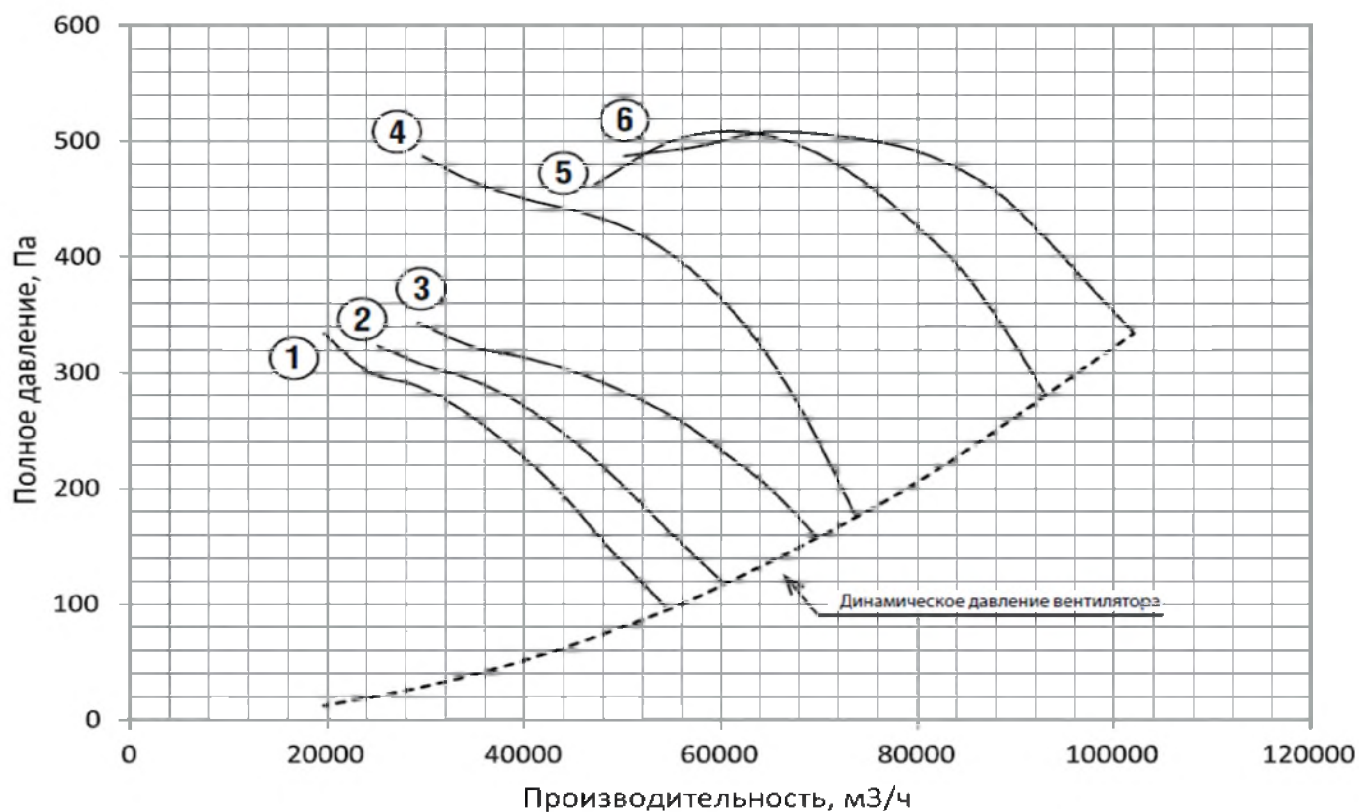
Рис. 13 Аэродинамическая характеристика AXIS №12,5 1000 об/мин
