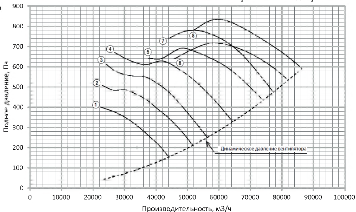
Рисунок 11. Аэродинамическая характеристика вентилятора AXIS №10 1500 об/мин
