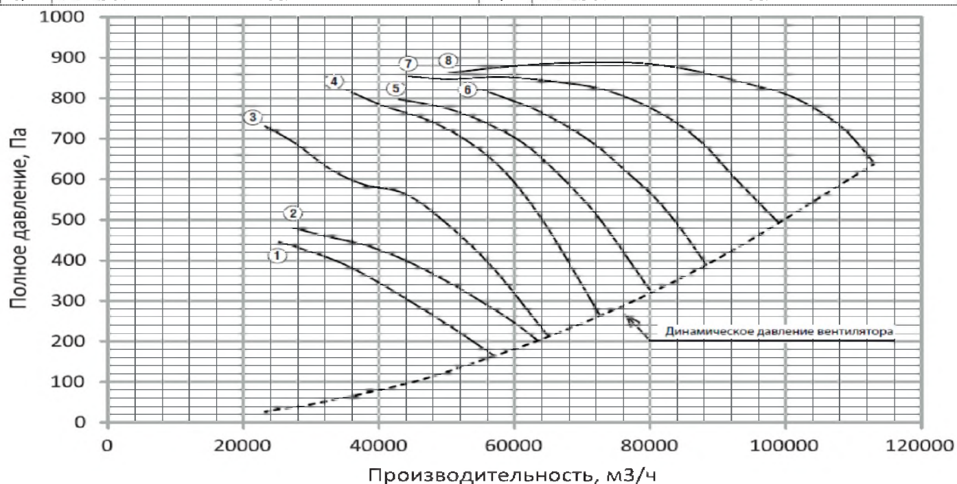
Рис 12. Аэродинамическая характеристика вентилятора AXIS №11,2 1500 об/мин.
