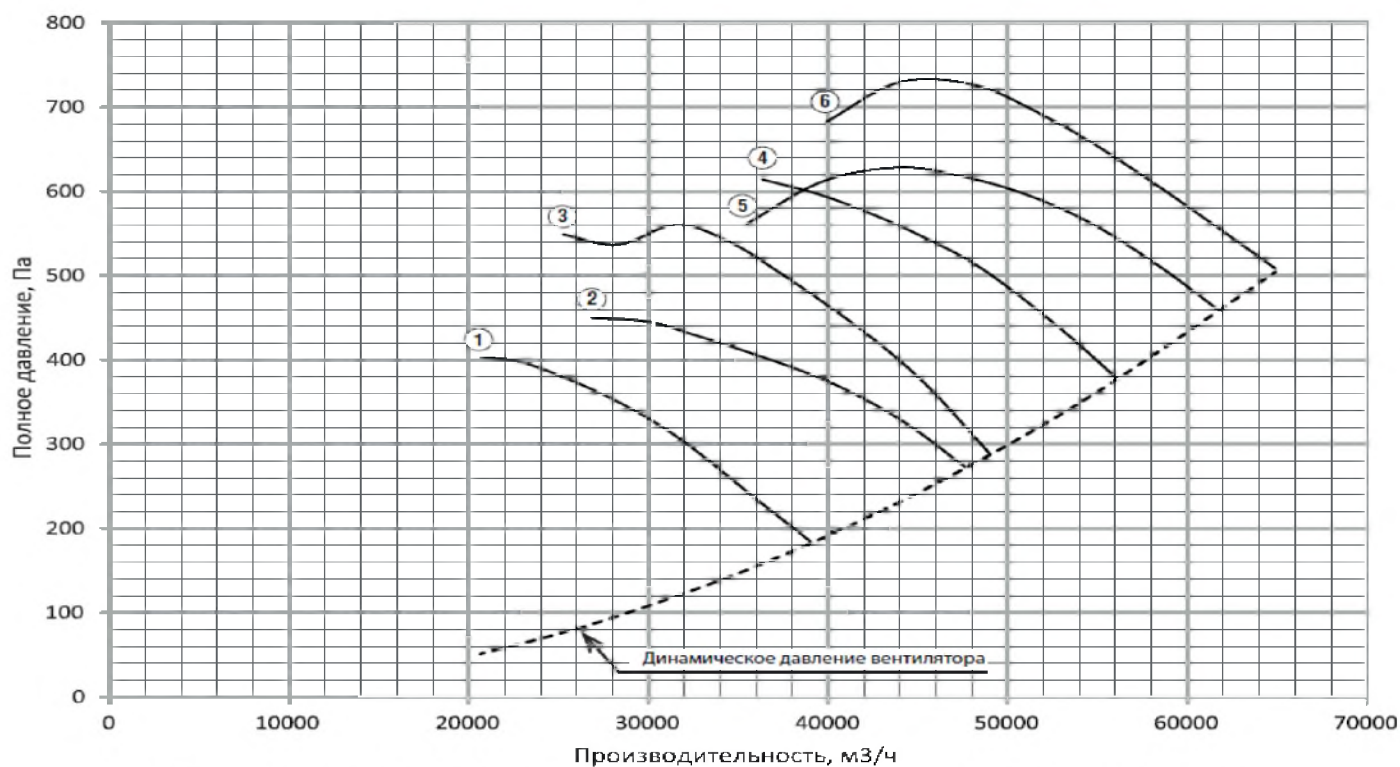
Рисунок 10. Аэродинамическая характеристика вентилятора AXIS №9 1500 об/мин
