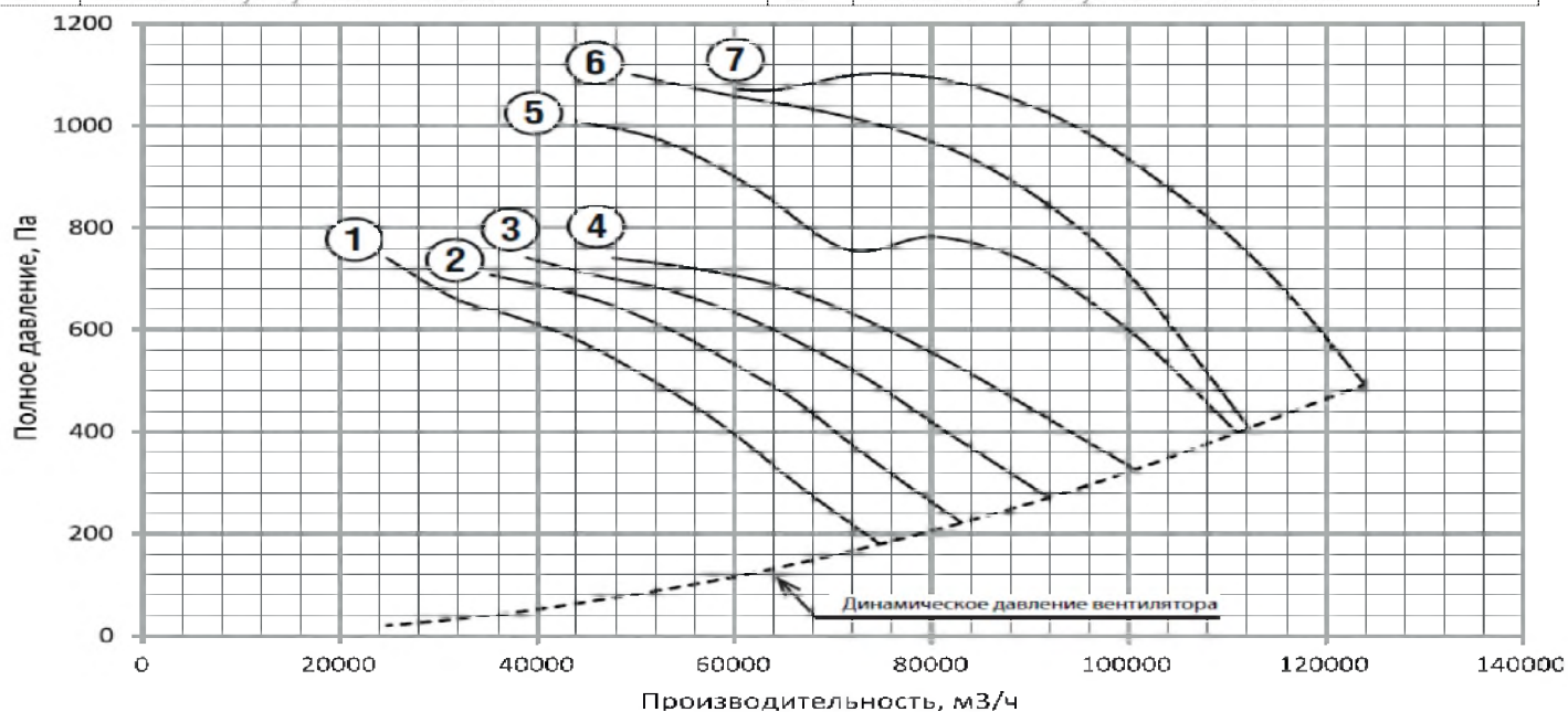
Рис. 14 Аэродинамическая характеристика AXIS №12,5 1500 об/мин
