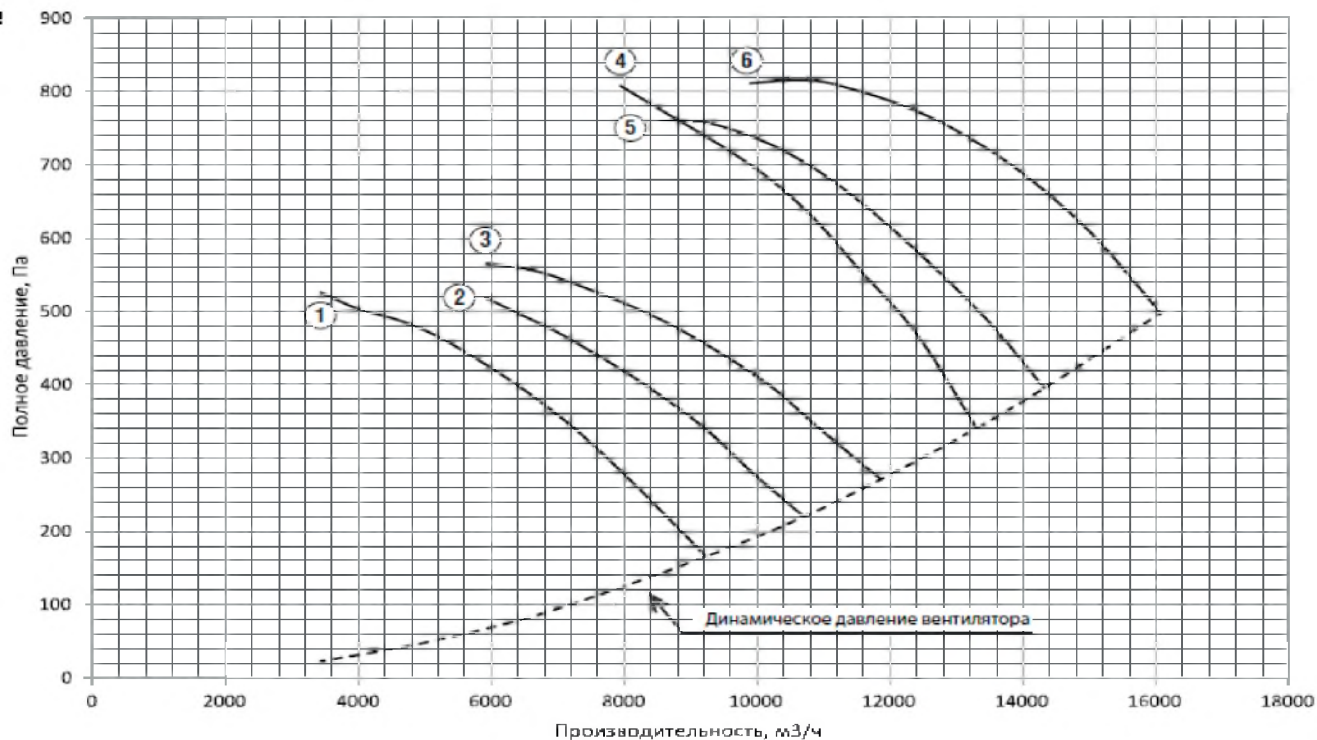
Рисунок 3. Аэродинамическая характеристика вентилятора AXIS №4,5
