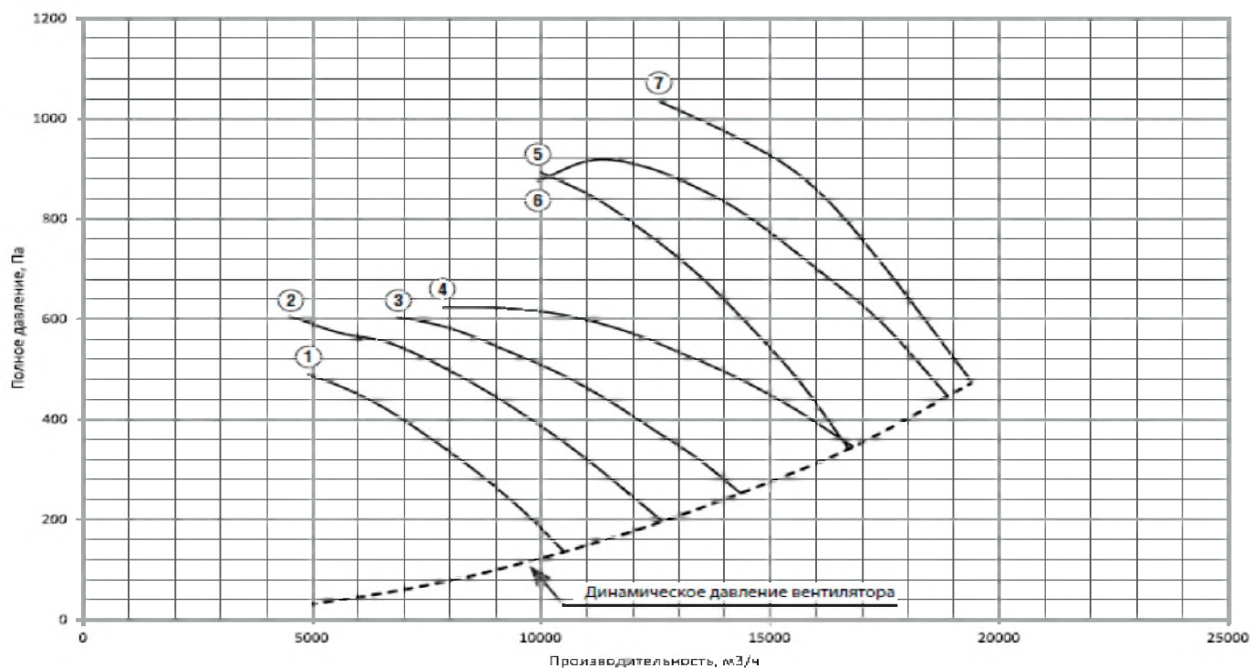
Рисунок 4. Аэродинамическая характеристика вентилятора AXIS №5
