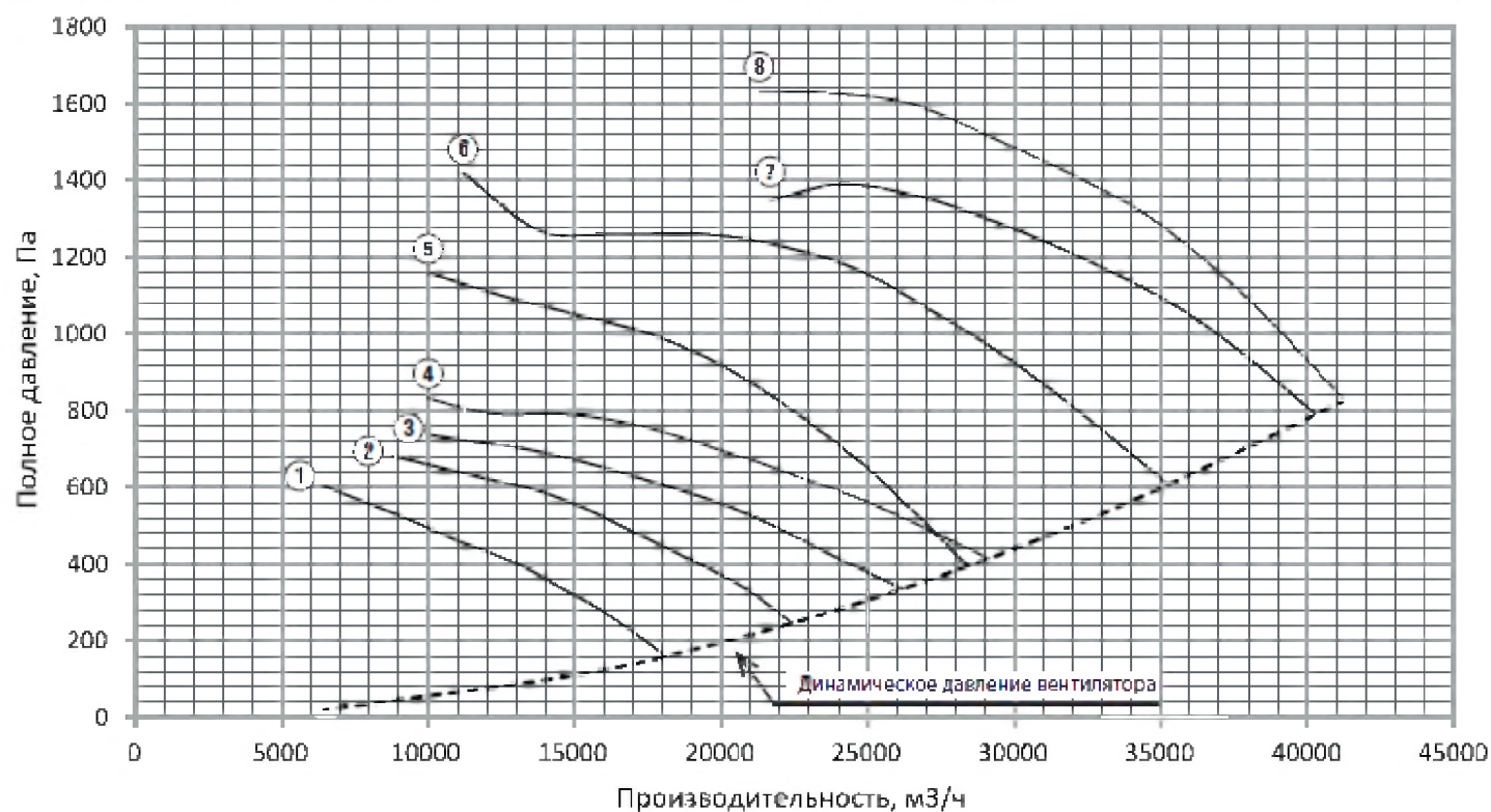
Рисунок 6. Аэродинамическая характеристика вентилятора AXIS №6,3
