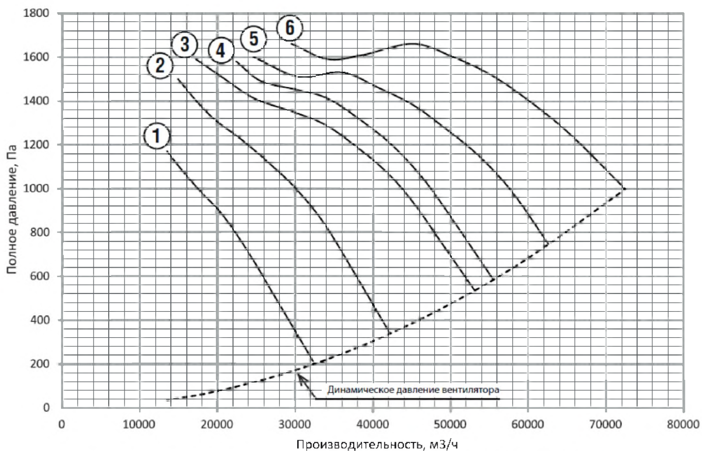
Рисунок 9. Аэродинамическая характеристика вентилятора AXIS №8 3000 об/мин
