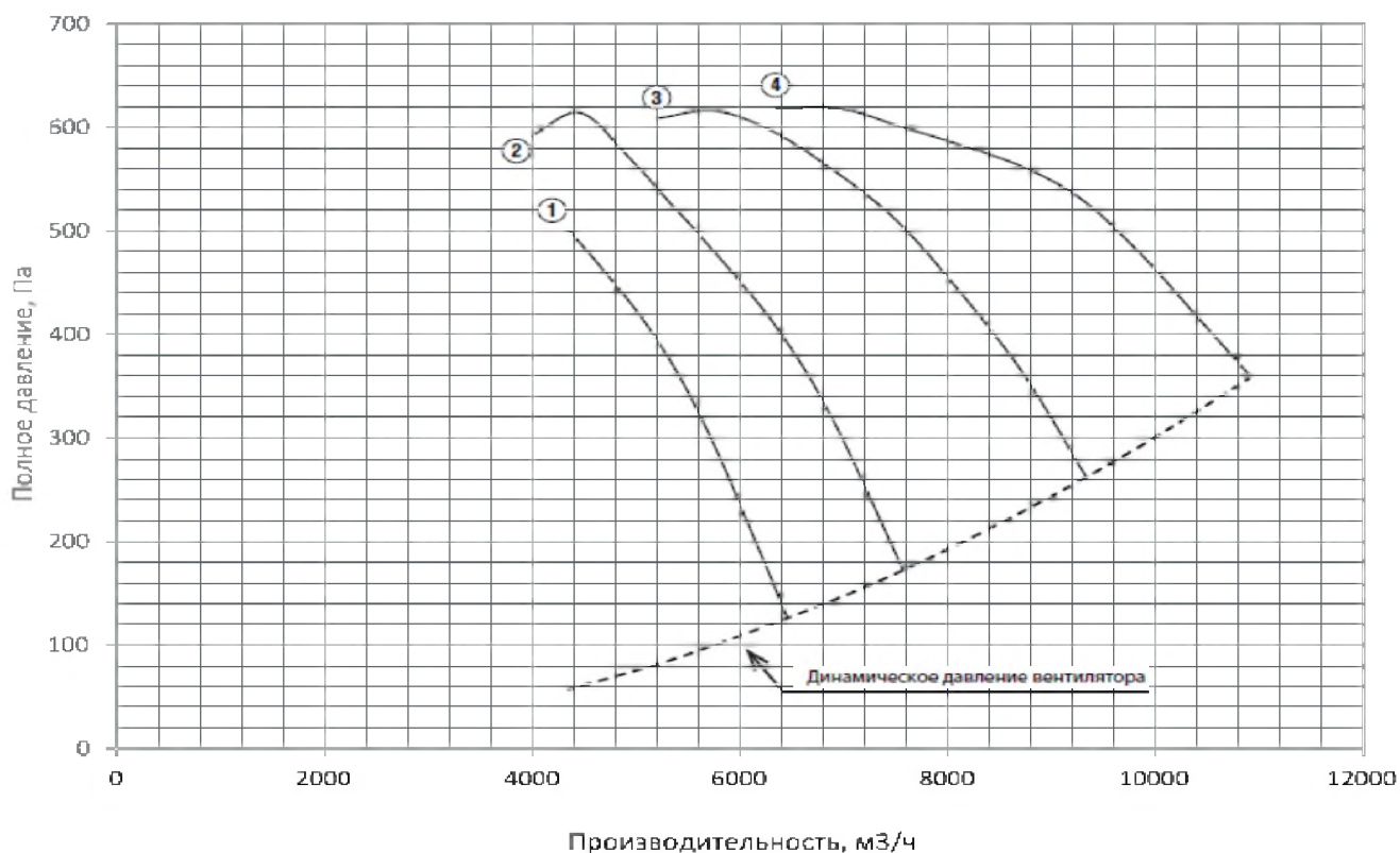
Рисунок 2. Аэродинамическая характеристика вентилятора AXIS №4
