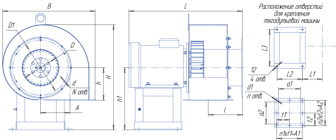
Габаритные и присоединительные размеры тягодутьевых машин ВД и Д №2,5; №2,7; №3,5.
