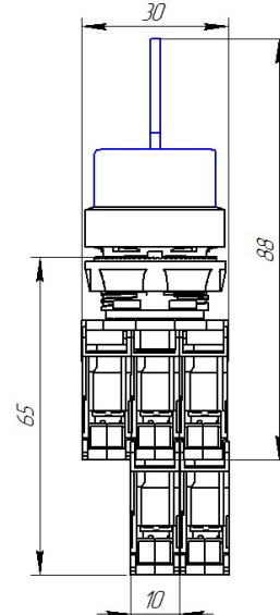
Рис.11. Переключатель с ключом.
