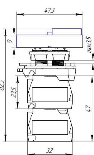
Рис.9. Кнопка двойная выступающая с пружинным возвратом.
