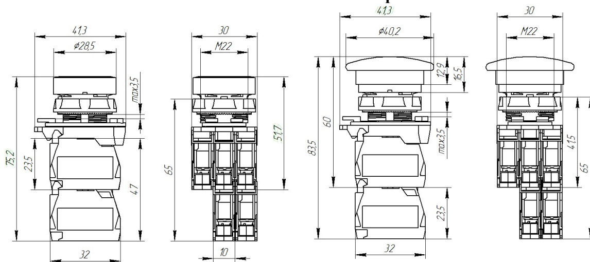
Рис.2. Выключатель кнопочный с цилиндрическим толкателем.
