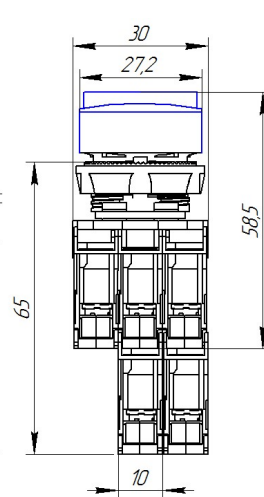
Рис.9. Кнопка двойная выступающая с пружинным возвратом.
