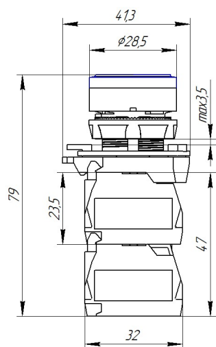
Рис.6. Выключатель кнопочный с подсветкой.
