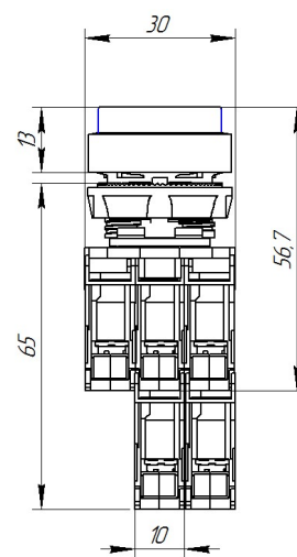
Рис.7. Выключатель кнопочный с выступающим цилиндрическим толкателем.
