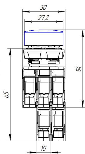
Рис.8. Кнопка двойная плоская с пружинным возвратом.
