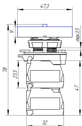
Рис.8. Кнопка двойная плоская с пружинным возвратом.
