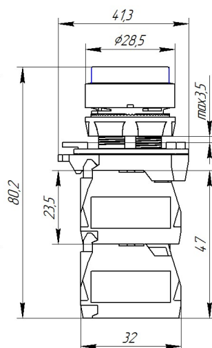
Рис.7. Выключатель кнопочный с выступающим цилиндрическим толкателем.
