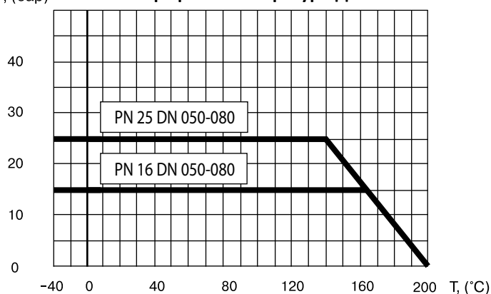
График «Температура-Давление»
