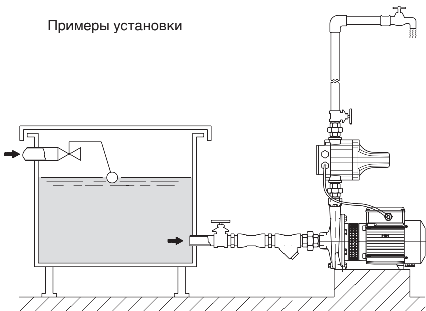
Fig. 1 Работа под гидравлическим напором
