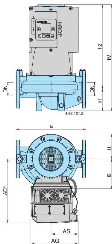
Фланцы PN 10, EN 1092-2
