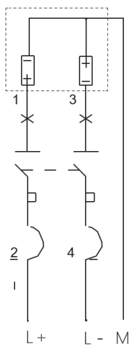
Подключение снизу
