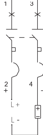
Подключение снизу
