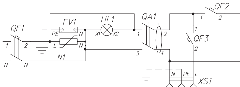
Рисунок 5. Схема ВРУ
