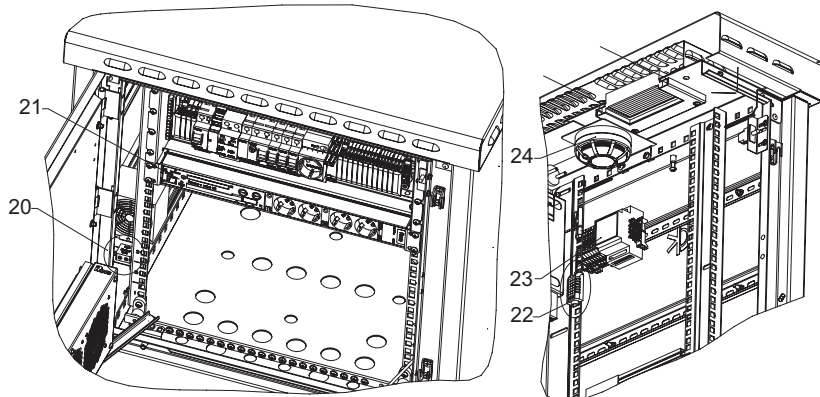
Рисунок 9. Контроллер МСх и датчики в шкафах ШТВ-1 и ШТВ-2
