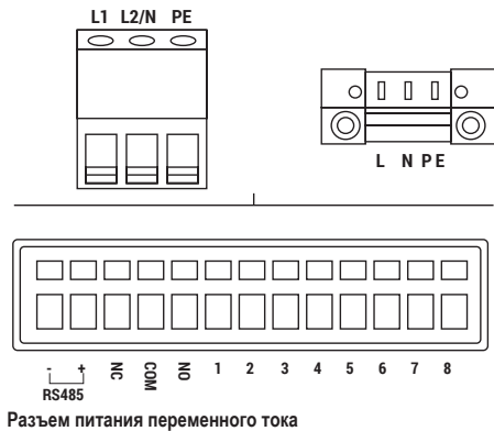
Рис. 2.1 Интерфейс подключения (данные о порте энергоснабжения содержатся в указаниях на заводской табличке с паспортными данными)
