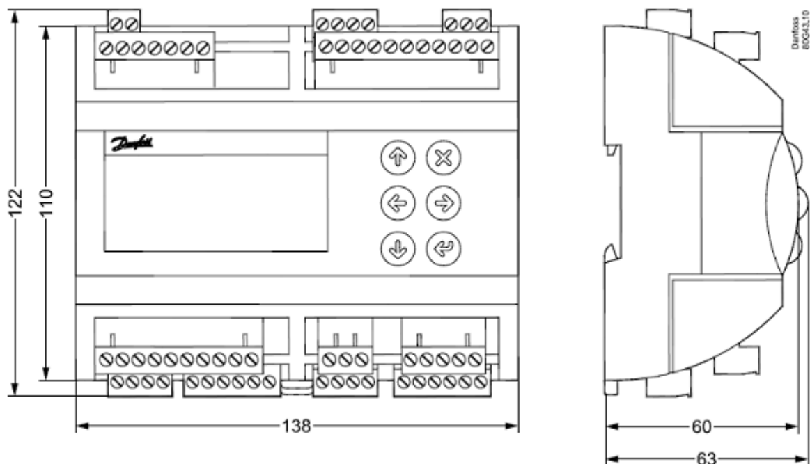
Контроллер давления и температуры типа АК-РС модификации 551
