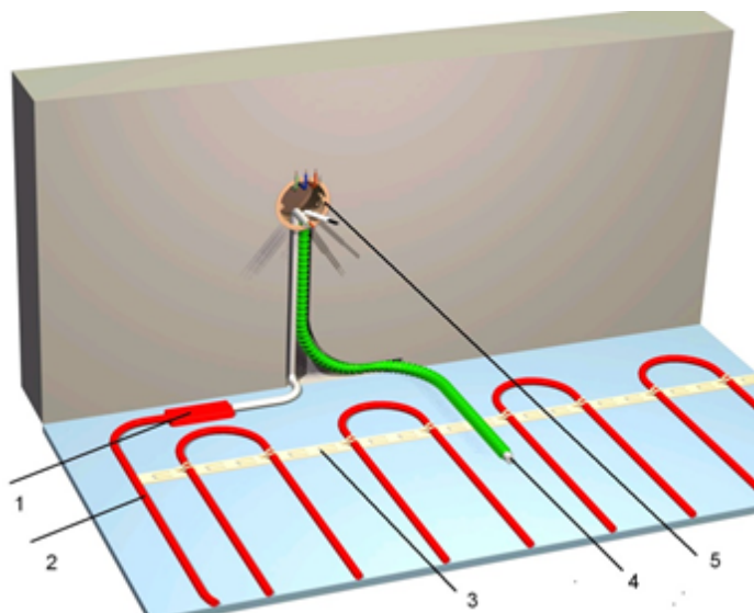
Рис. 3. Монтаж нагревательного кабеля DEVIflex™ 10T в бетонном полу.
