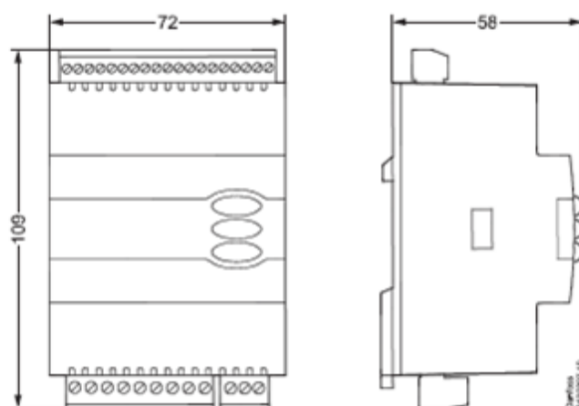
Габаритные размеры контроллеров типа ЕКС
