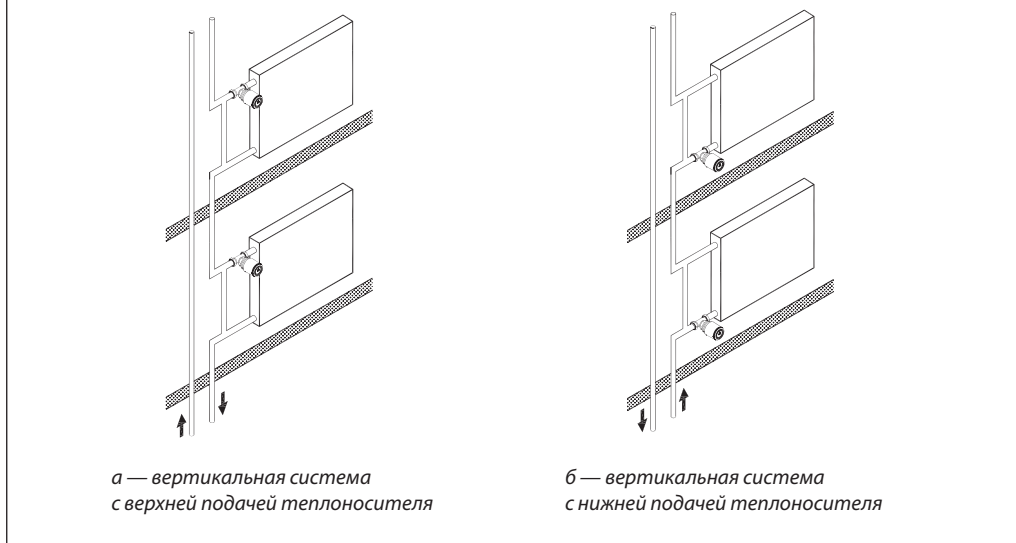
Одноконтурная насосная система отопления
