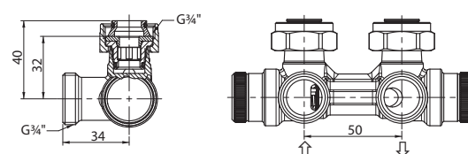
RLV-KDV угловой левый с присоединением к отопительному прибору G\frac{3}{4} "
