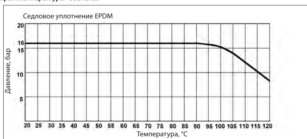
График температуры–давления
