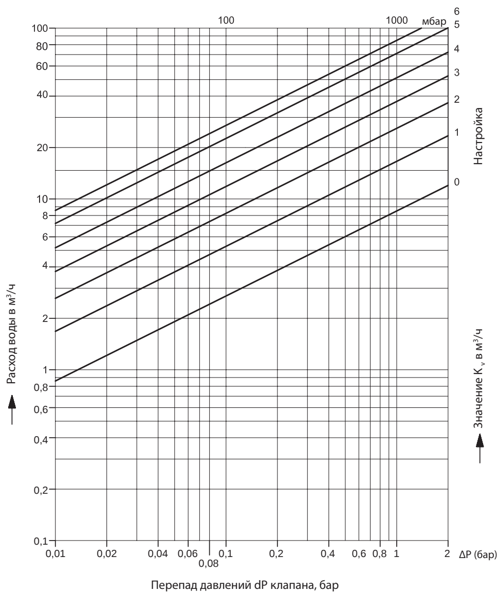
Расходная характеристика
