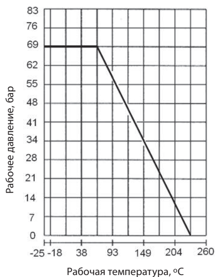
Кран шаровой стальной X1666, X2777
