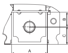
Размер монтажного отверстия клеммной пластины (единица измерения: мм)
