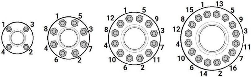
Рисунок 8 – Порядок затяжки крепежных болтов/шпилек
