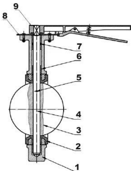
Рисунок 1 – Деталировка
