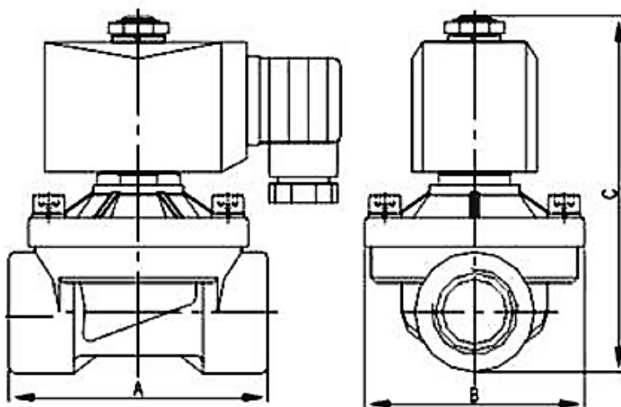
Рисунок 1 – Размеры
