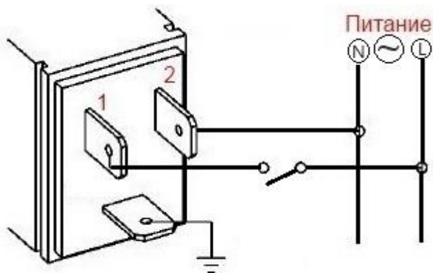
Рисунок 2 – Схема подключения на переменное напряжение
