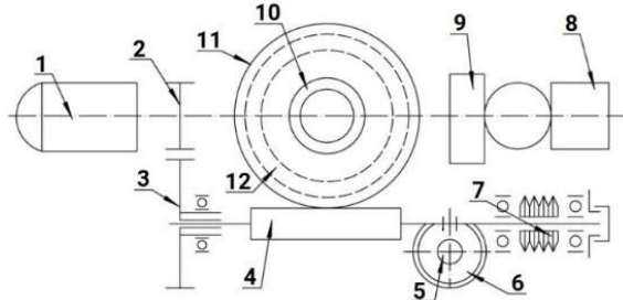
Рисунок 3 – Элементы электропривода
