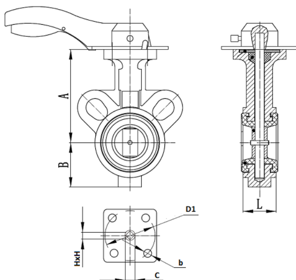
Рисунок 2 - Размеры
