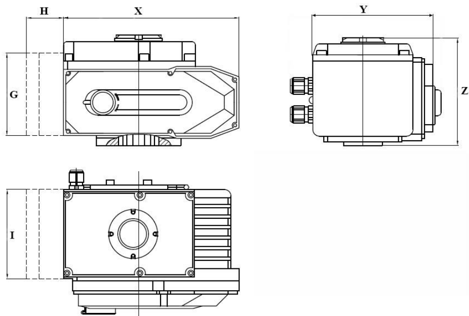
Рисунок 2 – Размеры приводов 030-040
