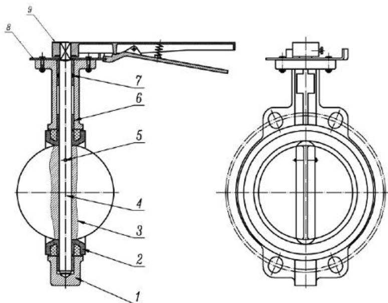
Рисунок 1. Деталировка
