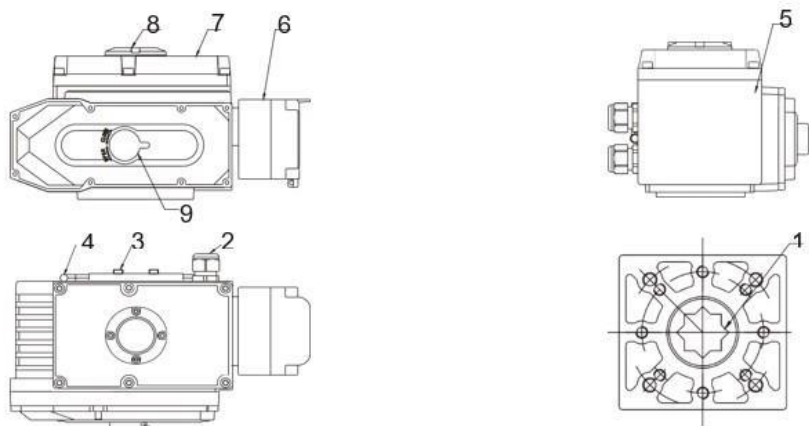
Рисунок 1 - Деталировка
