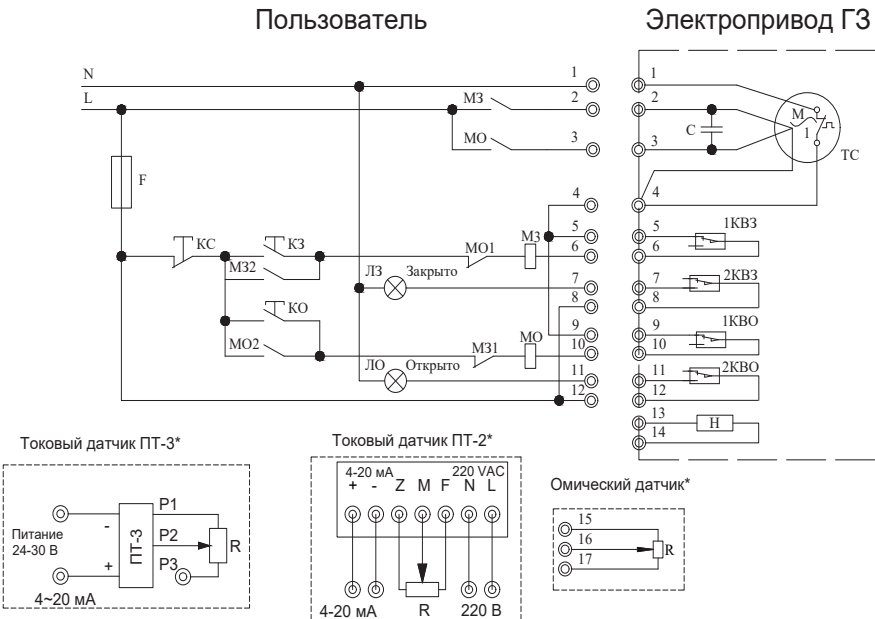
Рис. 2(1). Принципиальная электрическая схема для электроприводов ГЗ-ОФ(К) к сети 220В (230В), 50 Гц.
