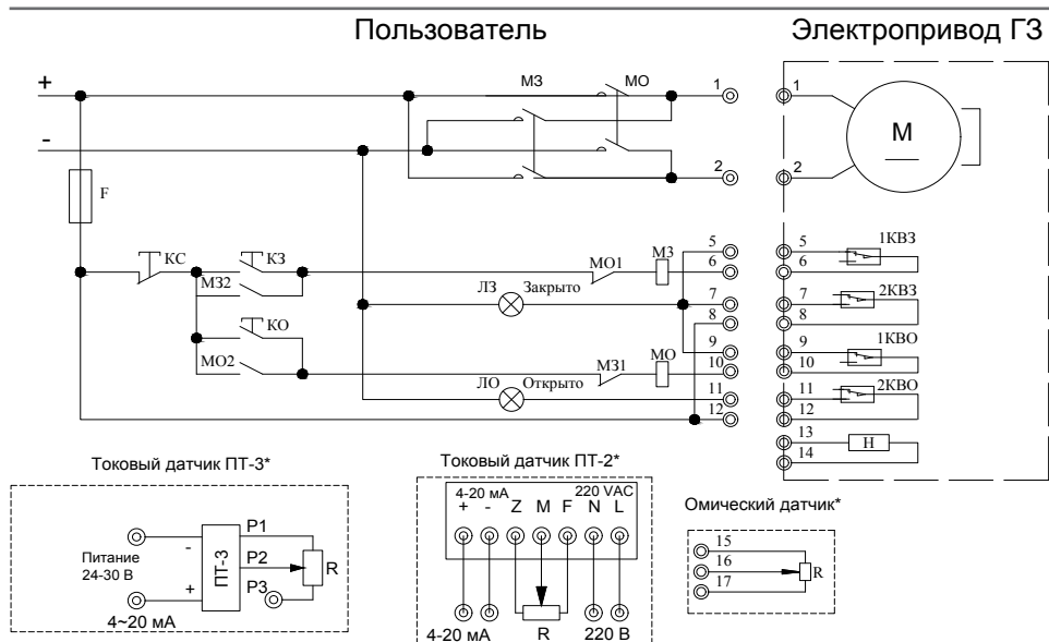
Рис. 2(3). Принципиальная электрическая схема для электроприводов ГЗ-ОФ(К) к сети 24В.
