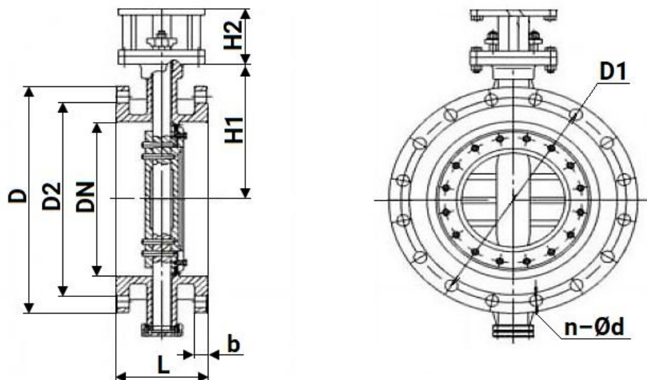
Рисунок 2 – Размеры
