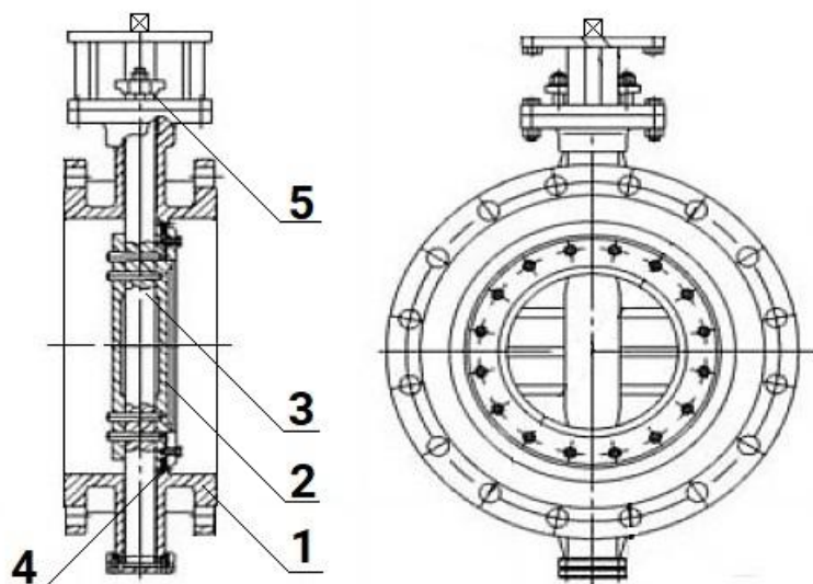
Рисунок 1 – Деталировка
