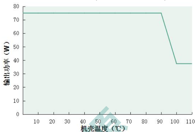
输出功率 VS 机壳温度(DL-75W-A/P-MXG)
