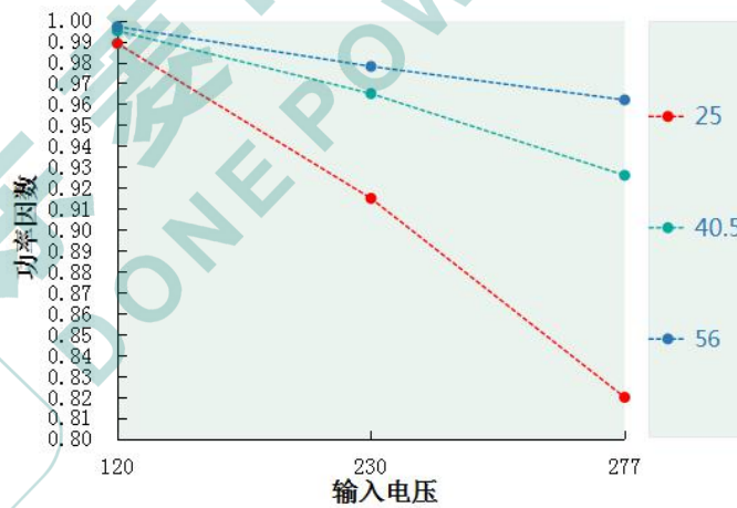
功率因素 VS 输入电压 DL-75W-V56A/P-MXG
