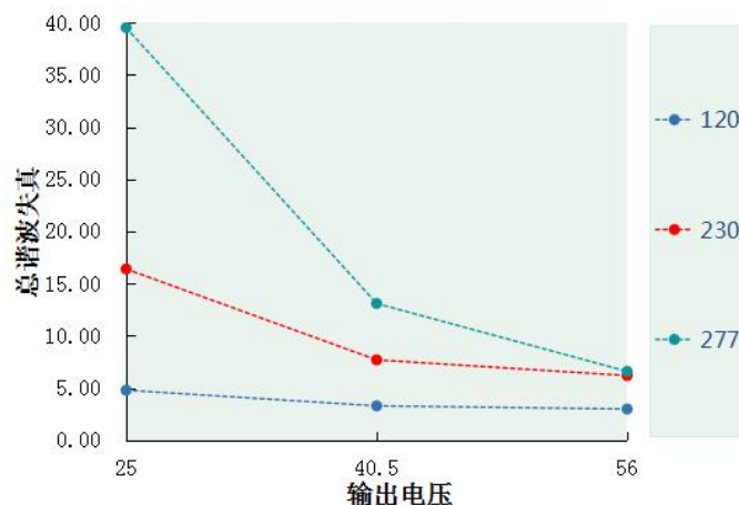
总谐波失真 VS 输出电压 DL-75W-V56A/P-MXG
