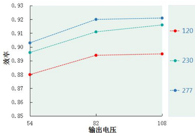
效率 VS 输出电压 DL-75W-V108A/P-MXG
