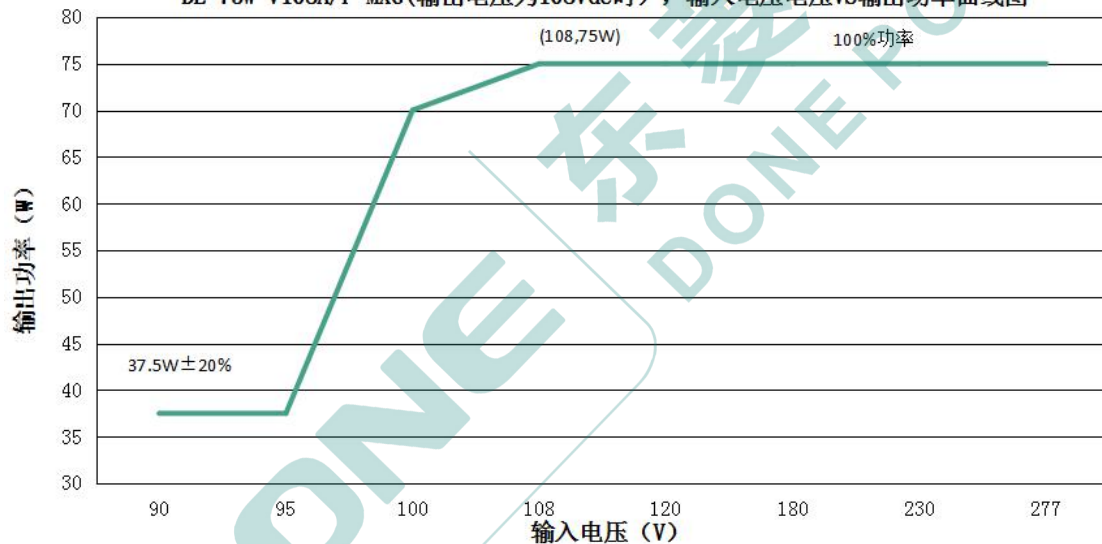
DL-75W-V108A/P-MXG(输出电压为108Vdc时), 输入电压电压VS输出功率曲线图
