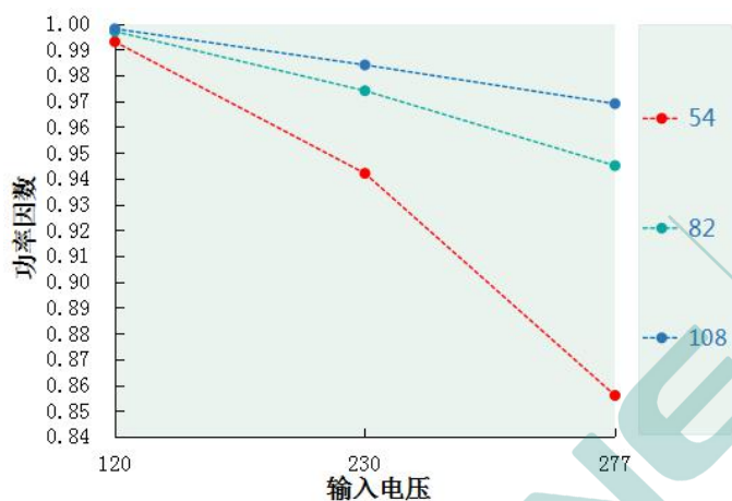
功率因素 VS 输入电压 DL-75W-V108A/P-MXG
