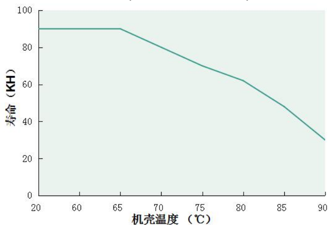
Tc VS 寿命(DL-75W-A/P-MXG)
