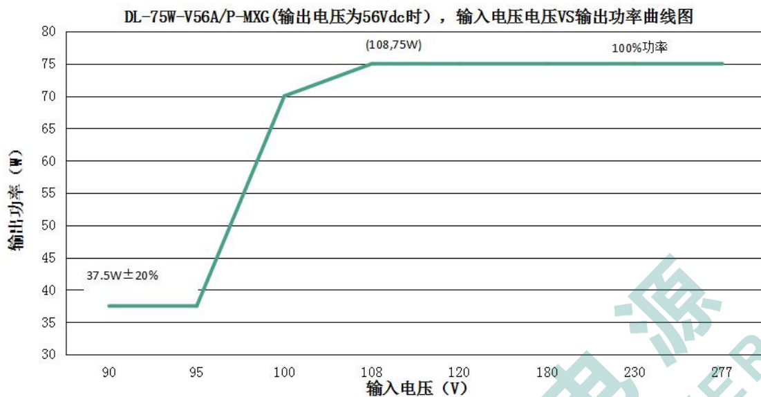
DL-75W-V56A/P-MXG(输出电压为 56Vdc 时，不同输入电压对应的额定输出电流值和输出功率)
