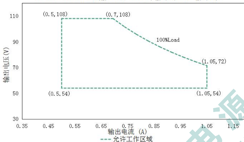
DL-75W-V108A/P-MXG(输入:120-277Vac)输出电压 VS 输出电流
