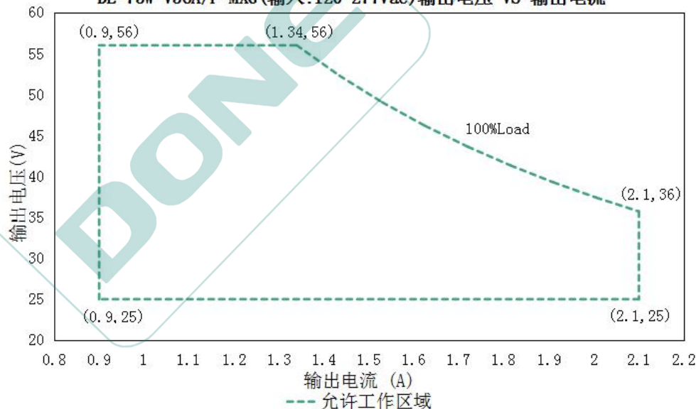
DL-75W-V56A/P-MXG(输入:120-277Vac)输出电压 VS 输出电流
