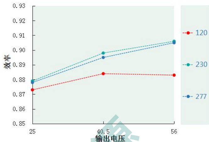
效率 VS 输出电压 DL-75W-V56A/P-MXG
