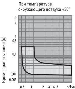
Рис. 2 – Время-токовые характеристики срабатывания дифференциальной защиты
