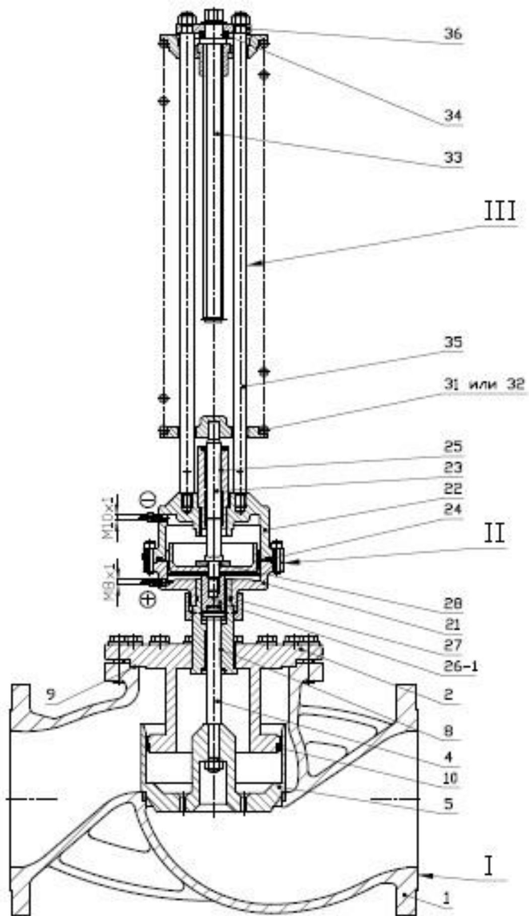
Рисунок 16- DN200
