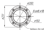
Фланец переходника для: 3ДВ 10-120, 3ДВ 10-160, 3ДВ 12-160, 3ДВ 12-240, 3ДВ 12-250
