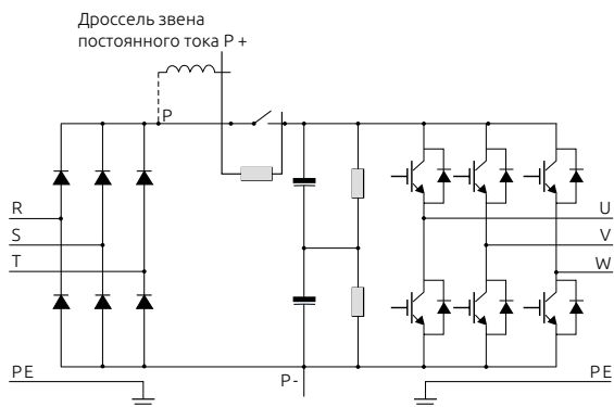
Рисунок 2-3. Схема силовой части (Больше 30кВт)
