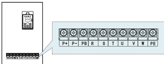
Рисунок 3-9. Схема силовых клемм ПЧ мощностью 11-18 кВт.
