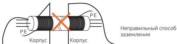
Рисунок 3-16. Схема заземления экрана
