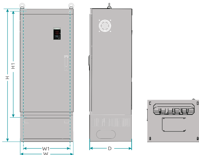
Рисунок 2-10. Установочные размеры ПЧ мощностью 200 — 560 кВт
