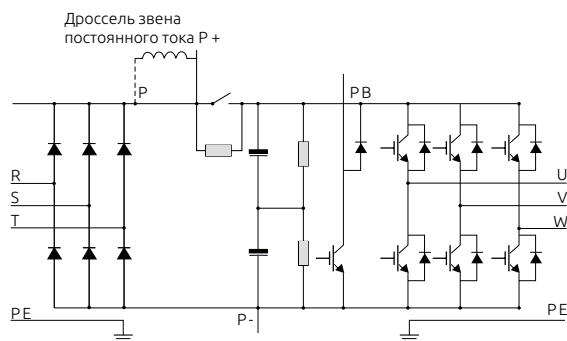
Рисунок 2-2. Схема силовой части (22кВт — 30кВт)
