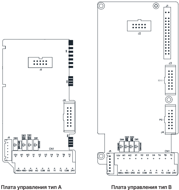
Рис. 3-10 Схема платы управления
