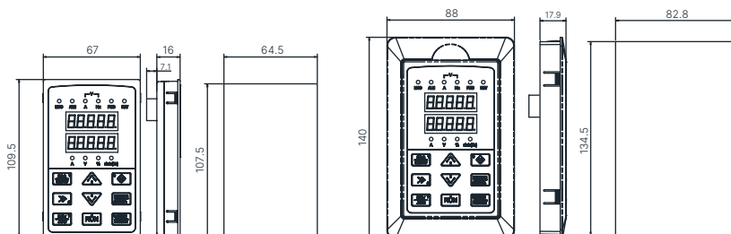
Рис. 2-5 EN-LED15 внешний вид и размеры отверстия клавиатуры
