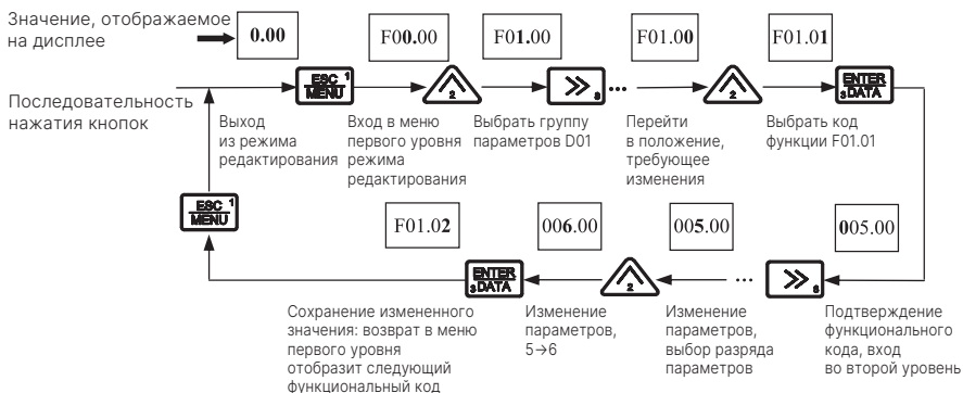
Рис. 5-8 Пример операций настройки и изменения параметров
