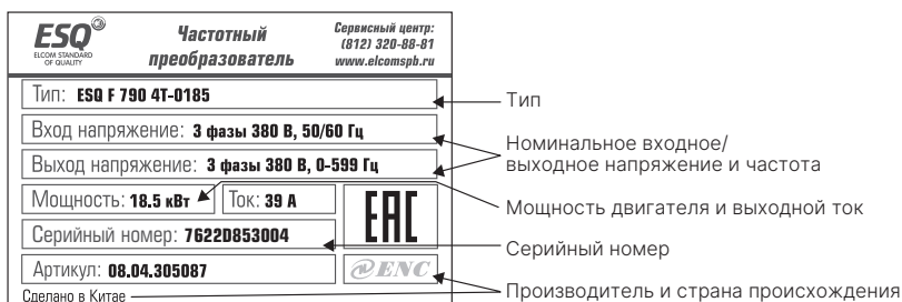
Рис. 2-2 Шильда
