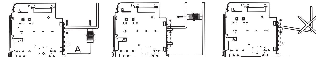
Крепление шинпровода
