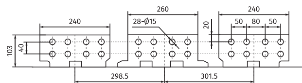
3 полюса
