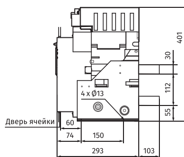
4 полюса
