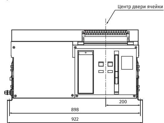
3 полюса
